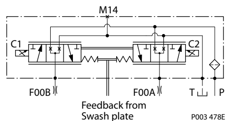
EDC 原理图，斜盘的反馈
