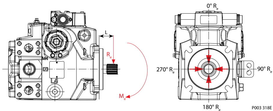
径向负载位置
