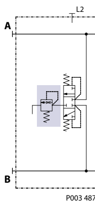
回路図
