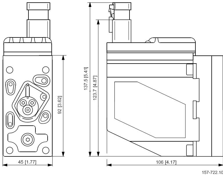
带 DEUTSCH 接头的 PVED-CC
