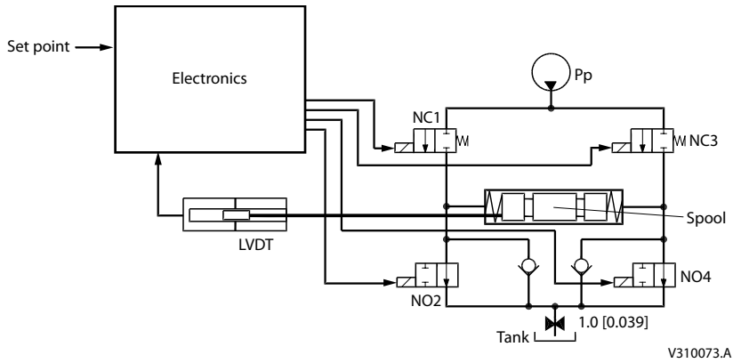
先导油简图
