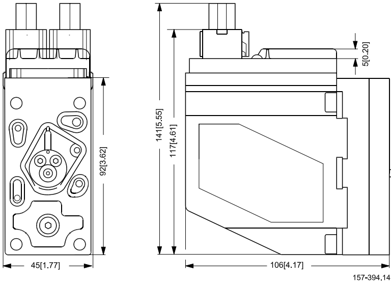
带 DEUTSCH 接头的 PVED-CC
