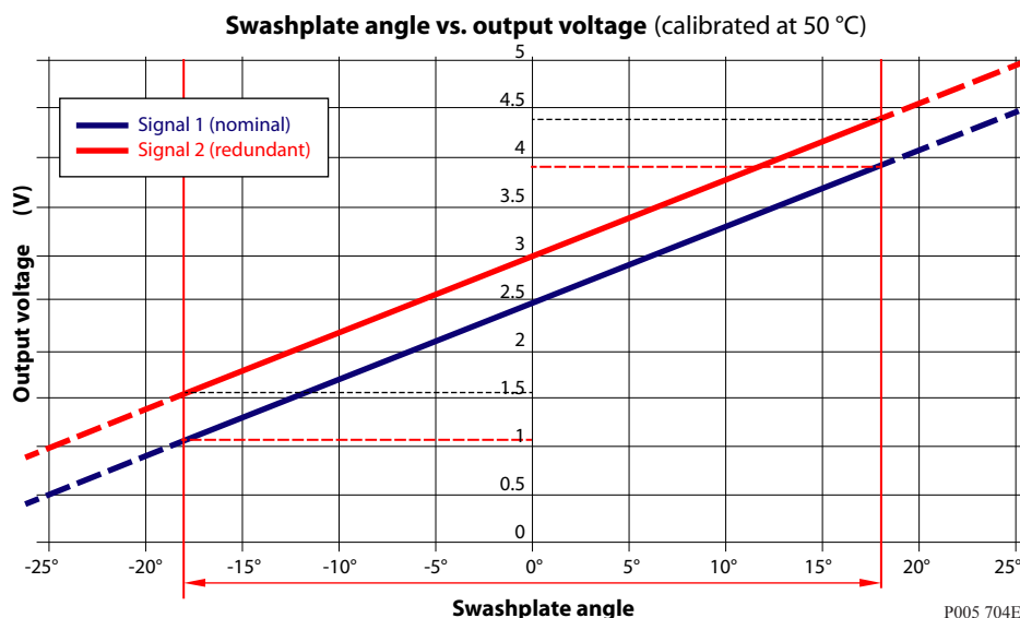
斜盘角度与输出电压
