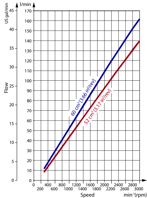
补油泵流量
