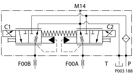
NFPE 原理图
