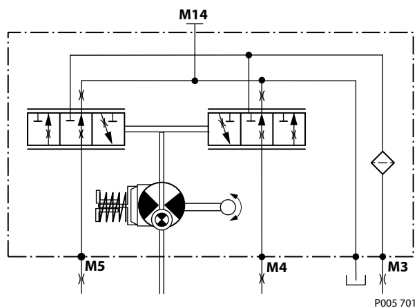
MDC 原理图
