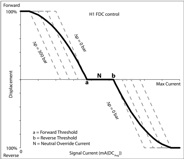
泵排量 vs. 控制电流
