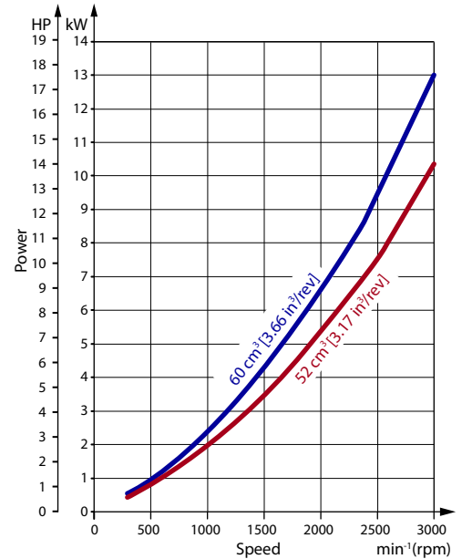
补油泵功率要求
