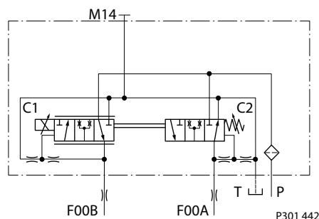
FDC 原理图
