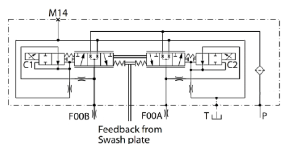
NFPE 回路図
