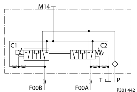
FDC 回路図
