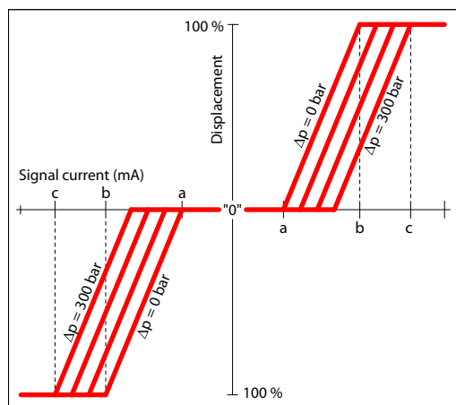
ポンプ容量と入力信号
