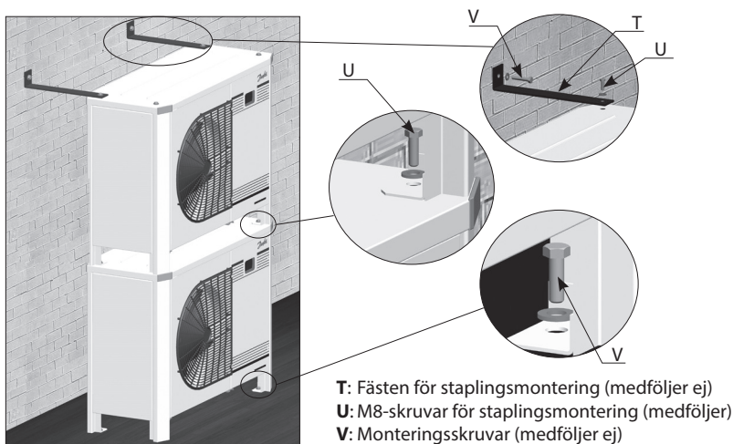
Bild 2: Staplingsmontering
