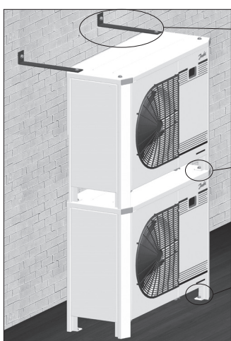
Figura 2: Montaggio a impilamento
