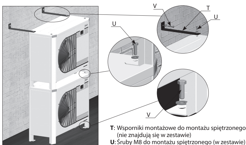
Rysunek 2: Montaż spiętrzony
