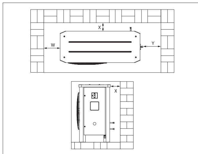
Bild 1: Minsta monteringsavstånd
