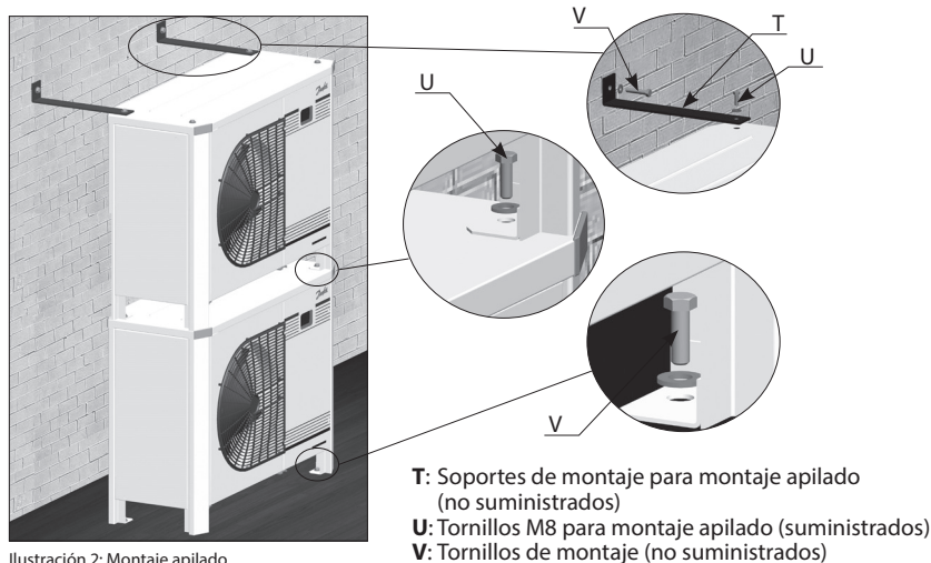
Ilustración 2: Montaje apilado
