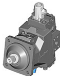
油圧アクチュエータ X1 加圧なし = 最小容量 フル加圧 = 最大容量
