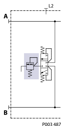
ループフラッシングリリーフバルブ (回路図)
