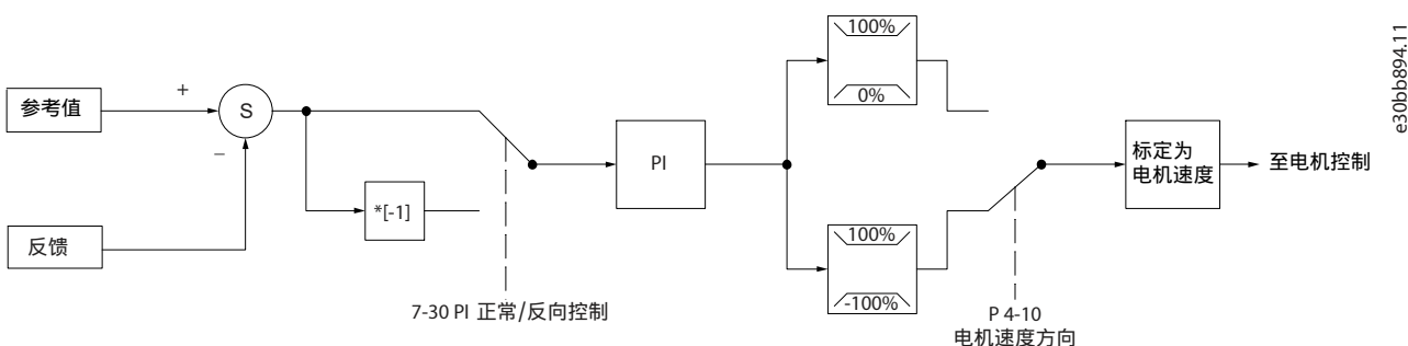
图 19: 闭环控制结构
