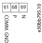
图 70: 网络连接
