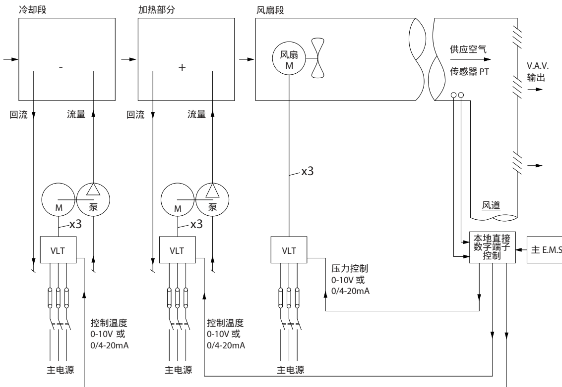
图 10: 由变频器控制的鼓风机系统
