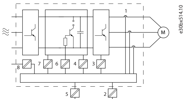
图 26: 电气隔离 110-315 kW (150-450 hp)
