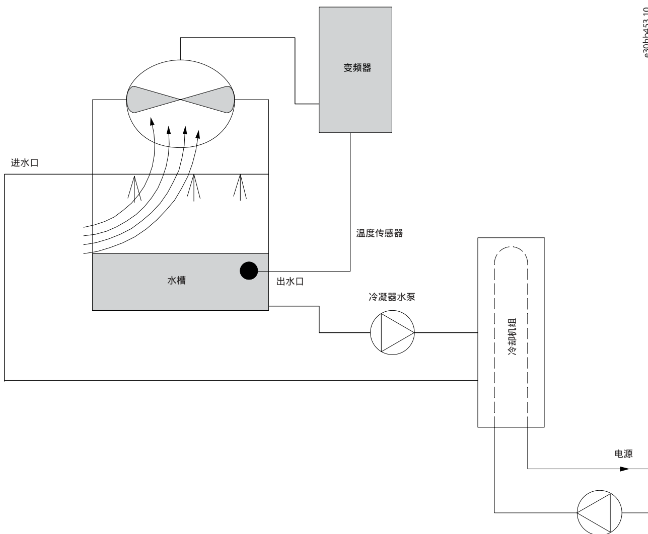
图 13: 冷却塔风扇
