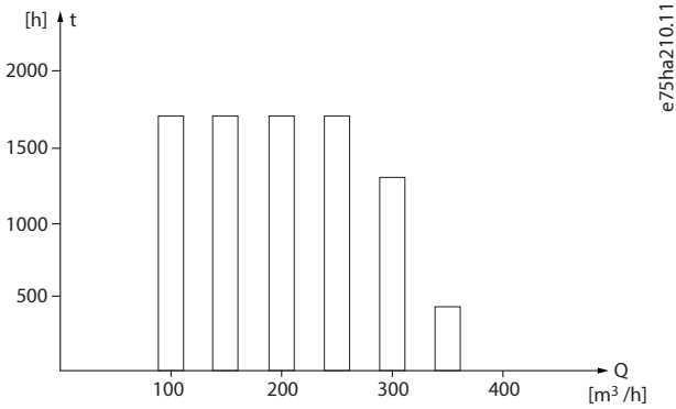
图 6: 一年的流量分布
