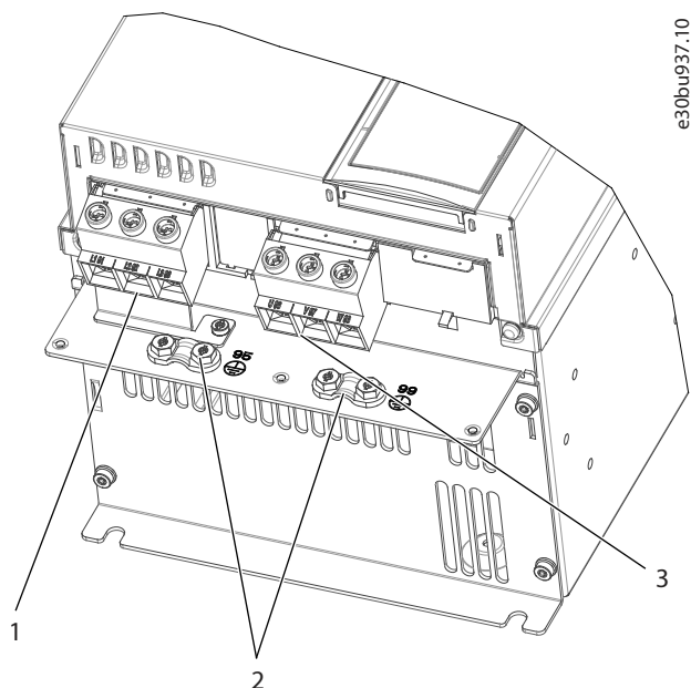
图 57: 机箱规格 H11、IP20、380-480 V、30-45 kW (40-60 hp)
