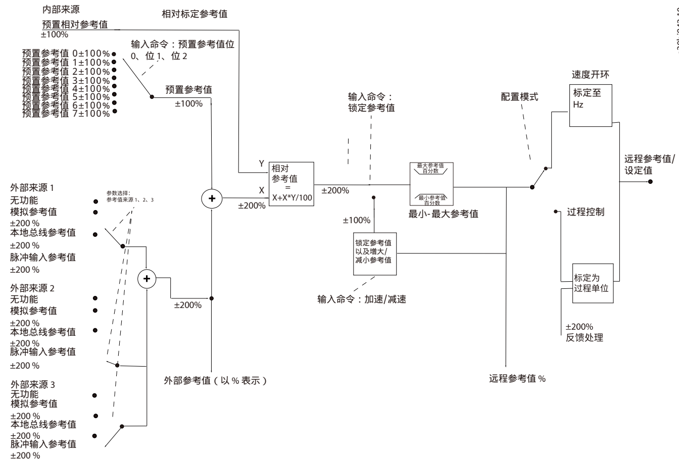
图 21: 框图显示了远程参考值
