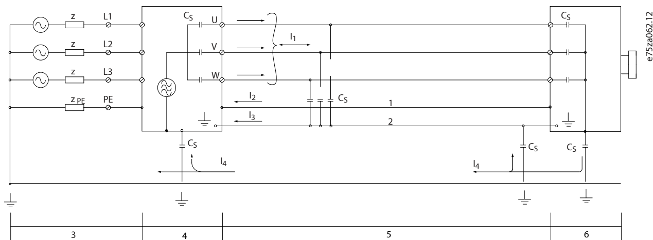
图 22: 漏电流的产生
