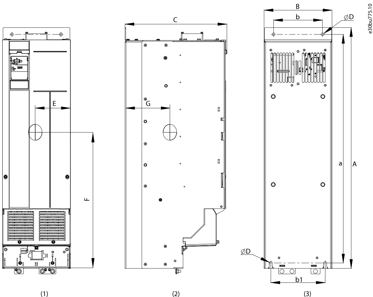
图 39: 机箱规格为 H13-H14 的变频器的尺寸
