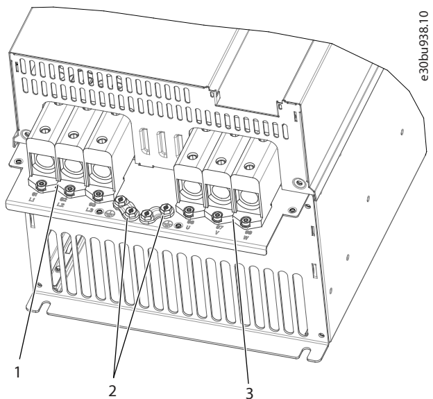
图 58: 机箱规格 H12、IP20、380-480 V、55-90 kW (75-125 hp)
