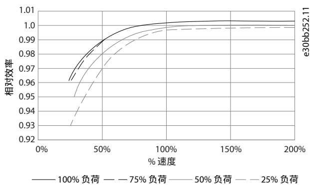
图 68: 典型效率曲线
