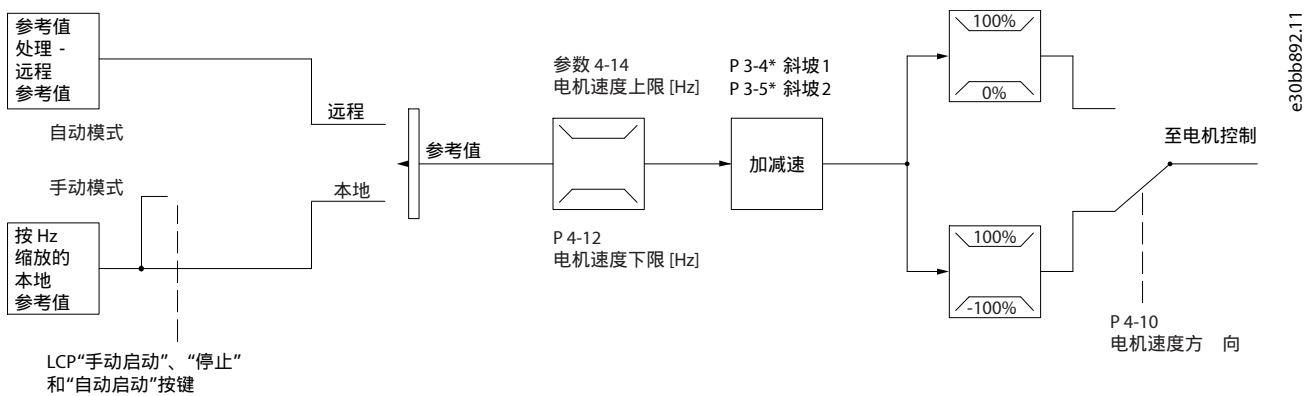
图 17: 开环结构
