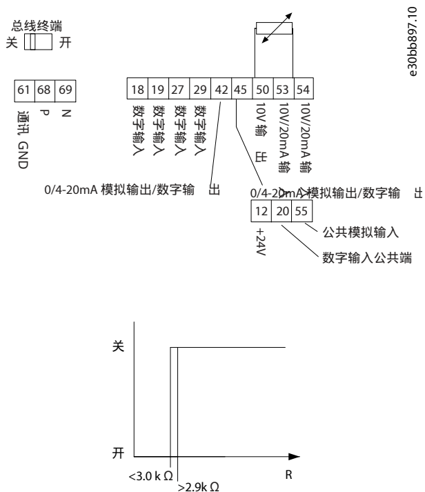
图 34: 模拟输入/10 V 电源
