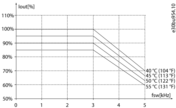
图 53: 110-315 kW (150-450 hp), 400 V, 机箱规格 H13-H14, IP20, 开关模式 SFAVM
