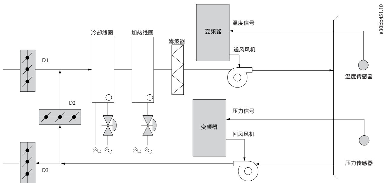
图 12: 定风量
