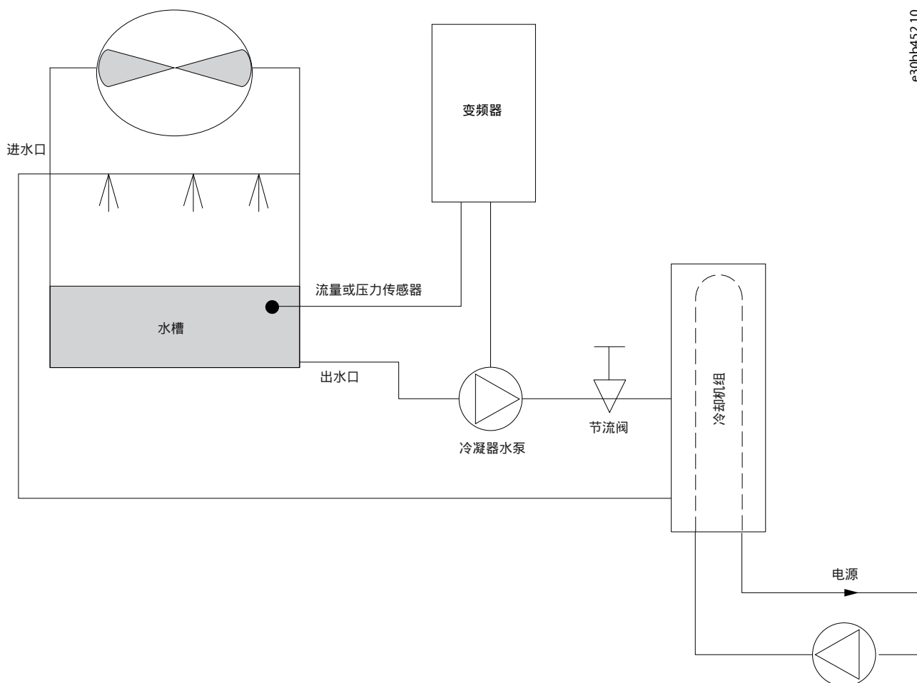
图 14: 冷凝器泵
