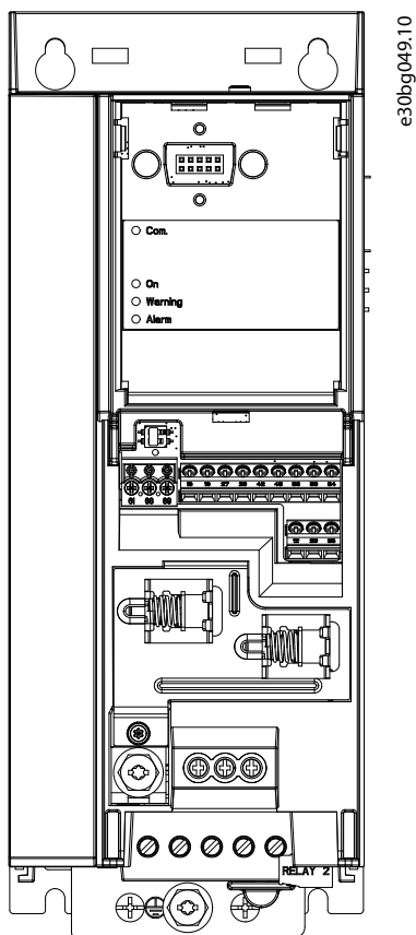
图 71: 终端电阻拨码开关的出厂设置
