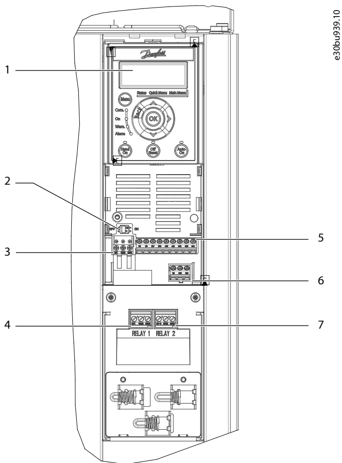
图 60: H11-H12 中的控制面板支架视图
