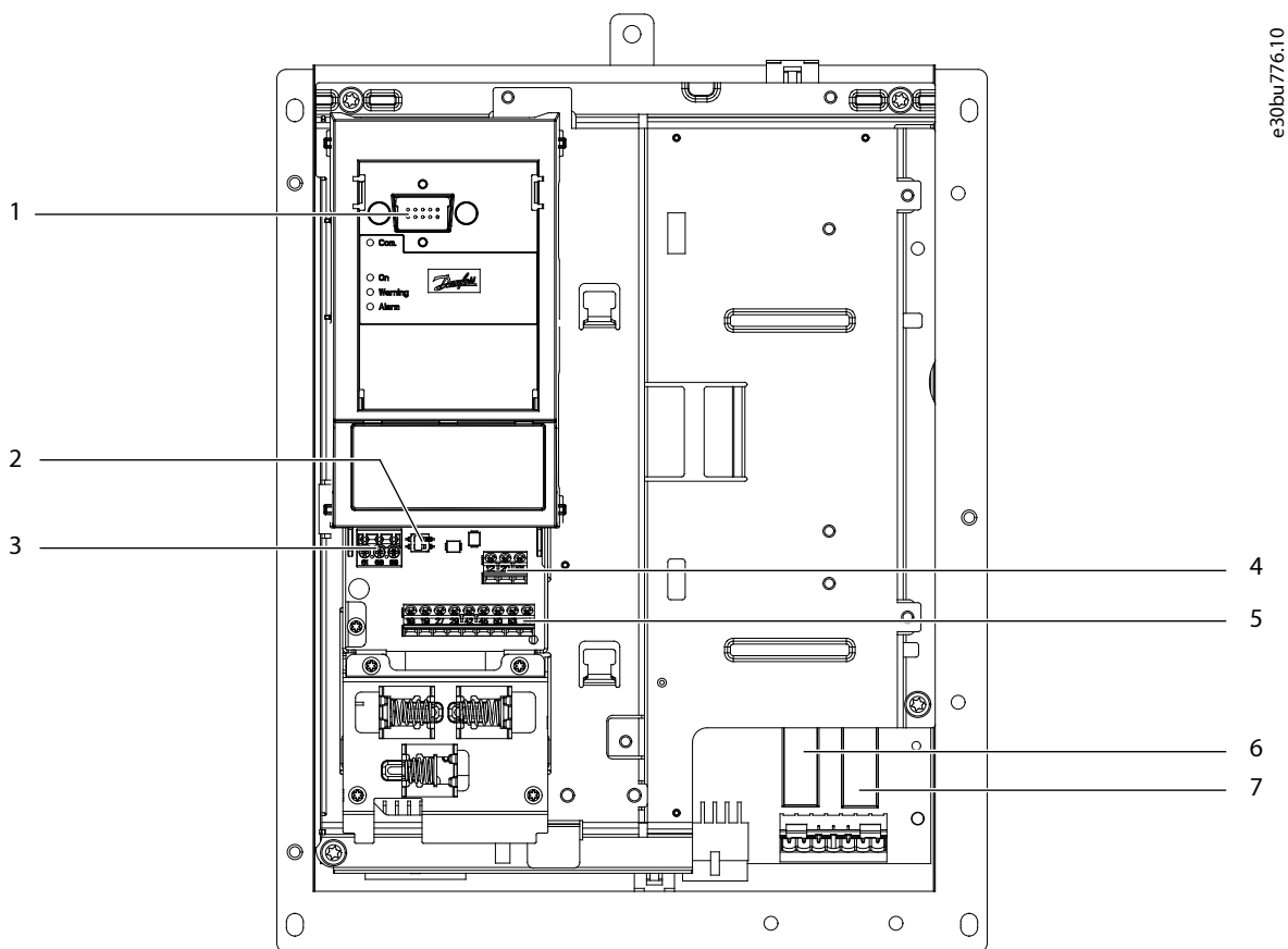
图 61: H13-H14 中的支架视图
