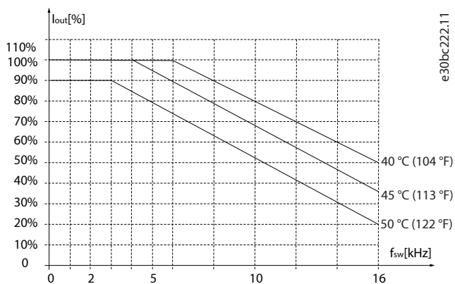
图 46: 5.5-7.5 kW (7.4-10 hp), 400 V, 机箱规格 H3, IP20
