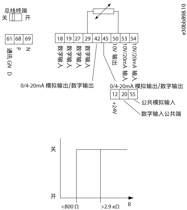
图 33: 数字输入/10 V 电源
