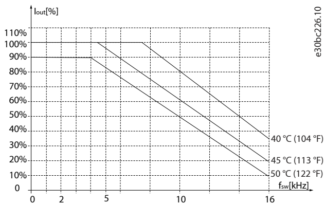
图 48: 18.5-22 kW (25-30 hp), 400 V, 机箱规格 H5, IP20
