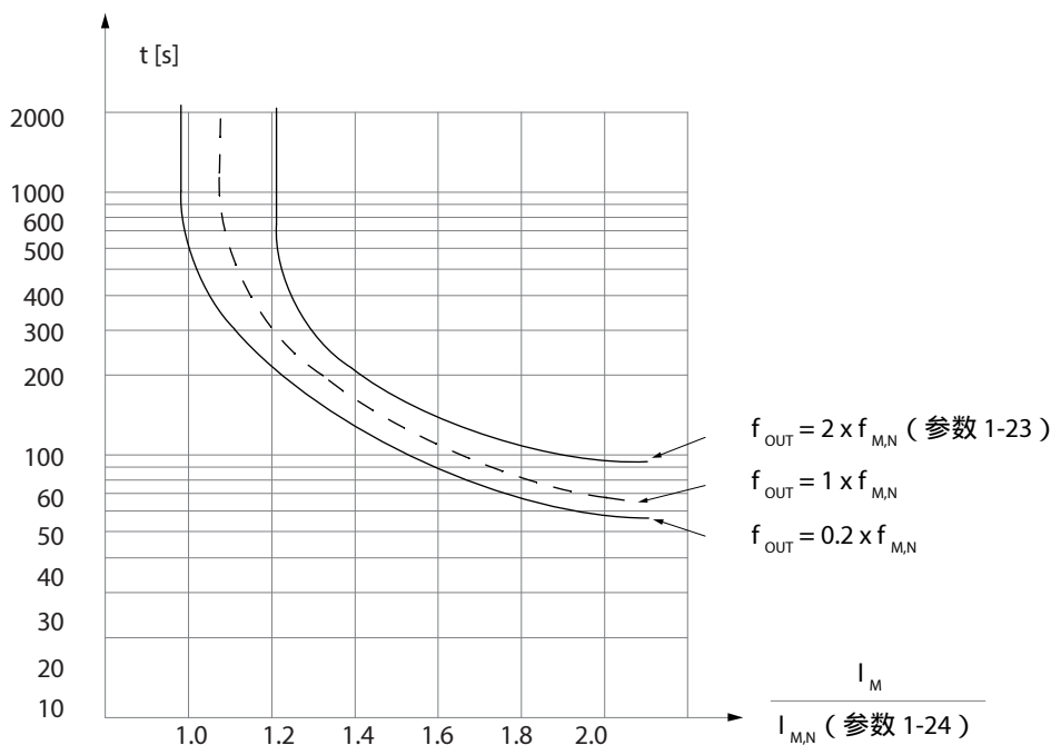
图 31: 电机热保护特性
