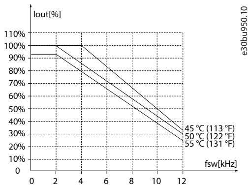
图 49: 30-45 kW (40-60 hp), 400 V, 机箱规格 H11, IP20
