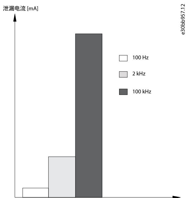
图 30: RCD 的截止频率对做出的响应/执行的测量的影响
