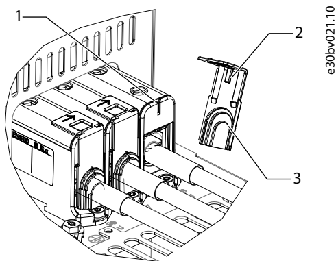
图 64: 安装保护盖, H12
