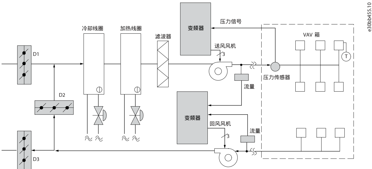
图 11: 变风量
