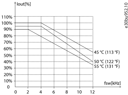
图 51: 90 kW (125 hp), 400 V, 机箱规格 H12, IP20
