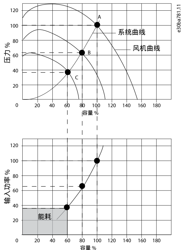
图 2: 通过变频器解决方案实现节能
