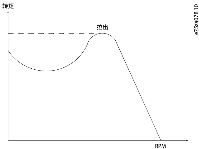
图 88: 起步转矩
