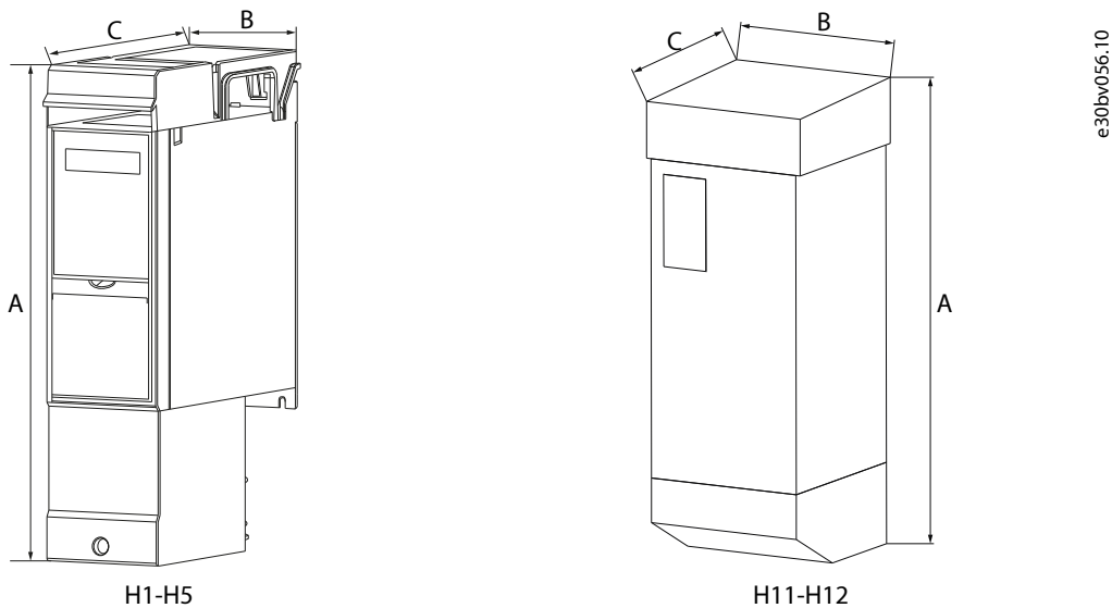
图 40: 机箱规格为 H1-H5 和 H11-H12 且带 IP21/ 类型 1 转换套件的变频器的尺寸
