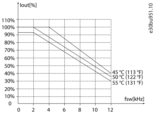
图 50: 55-75 kW (70-100 hp), 400 V, 机箱规格 H12, IP20
