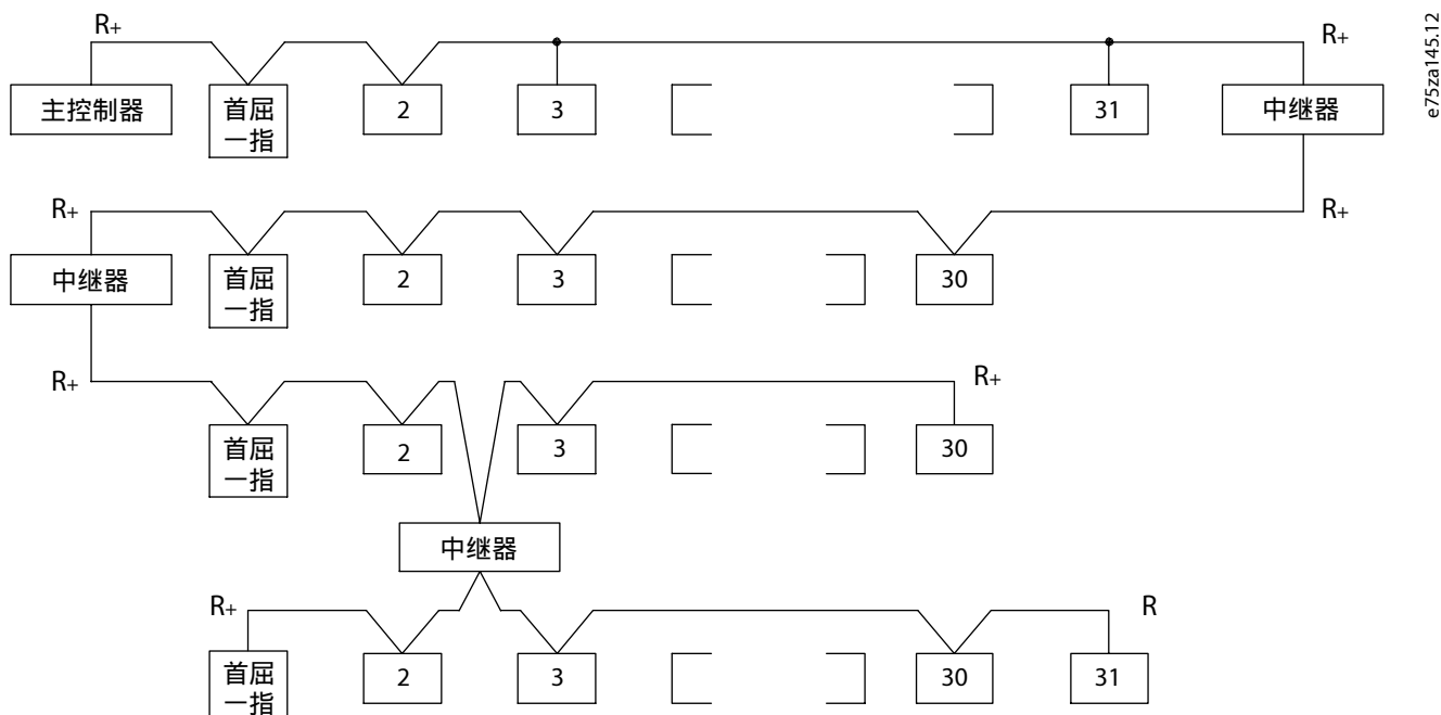
图 69: RS 485 总线接口
