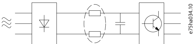
图 23: 直流回路电抗
