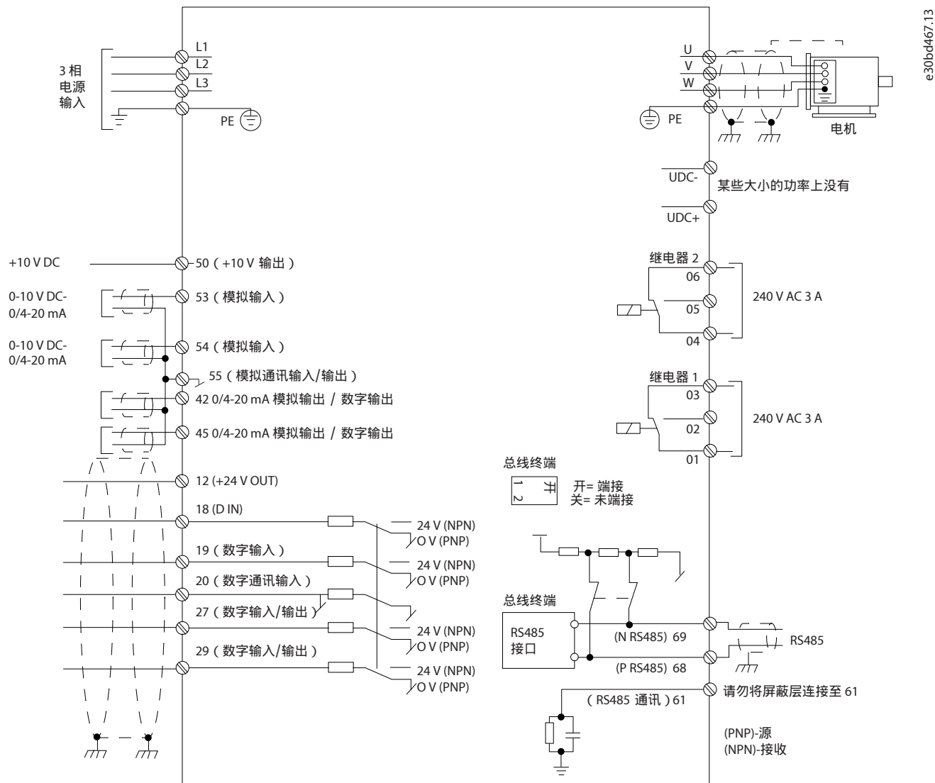
图 54: 基本接线示意图
