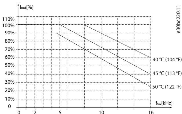
图 45: 2.2–4.0 kW (3.0–5.4 hp), 400 V, 机箱规格 H2, IP20
