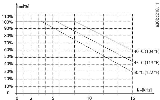
图 44: 0.37–1.5 kW (0.5–2.0 hp), 400 V, 机箱规格 H1, IP20
