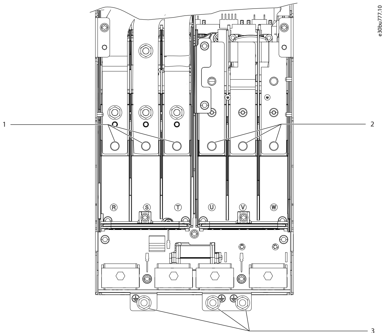
图 59: 机箱规格 H13-H14 IP20, 380-480 V, 110-315 kW (150-450 hp)
