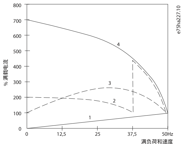
图 8: 启动电流
