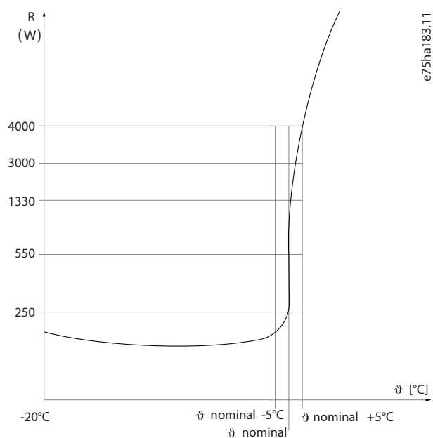
图 32: 电机温度过高时, 变频器将跳闸
