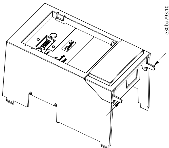
图 66: 拆除托架盖
