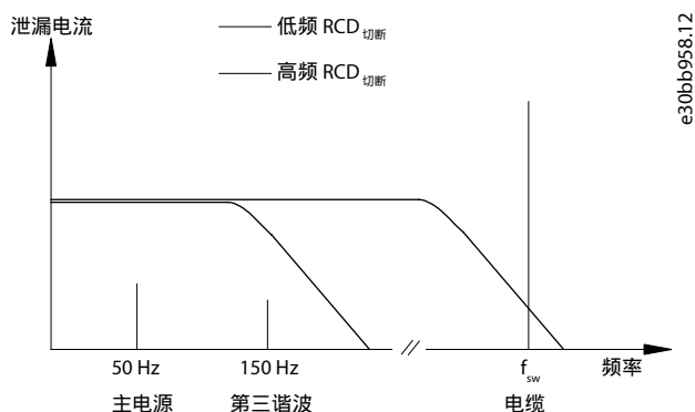
图 29: 主电源造成泄漏电流
