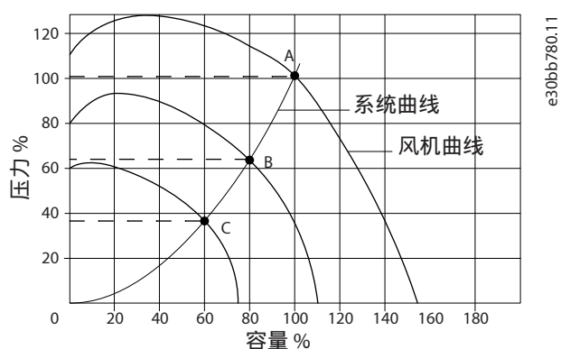
图 1: 降低风扇流量时的风扇曲线 (A、B 和 C)
