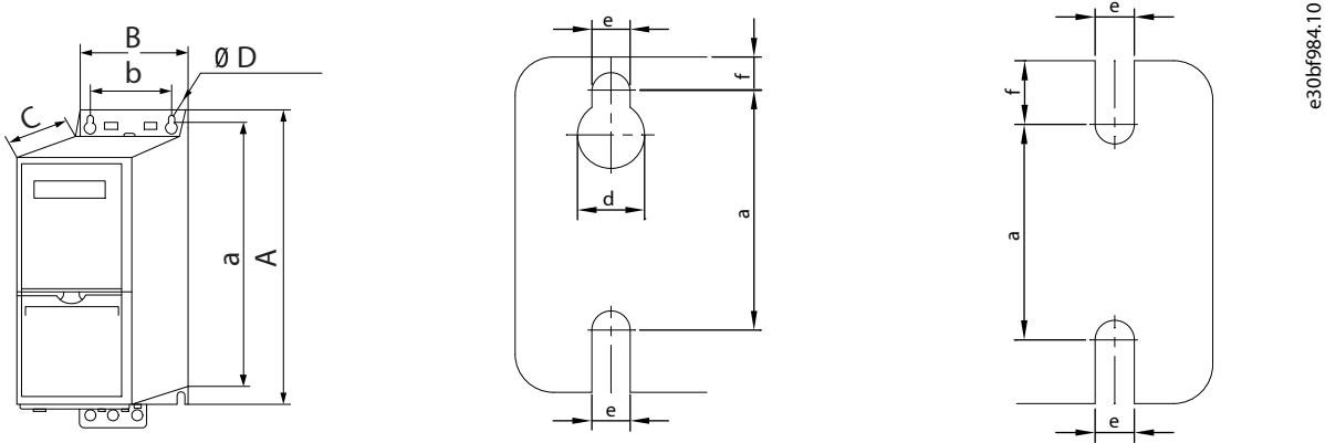
图 37: 机箱规格为 H1–H5 和 H11–H12 的变频器的尺寸
