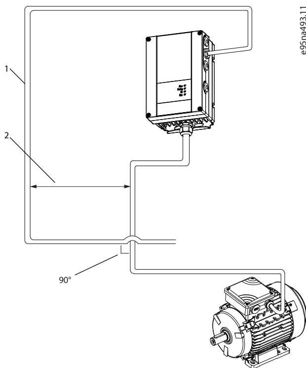
图 72: 通信电缆与电源电缆之间的最短距离
