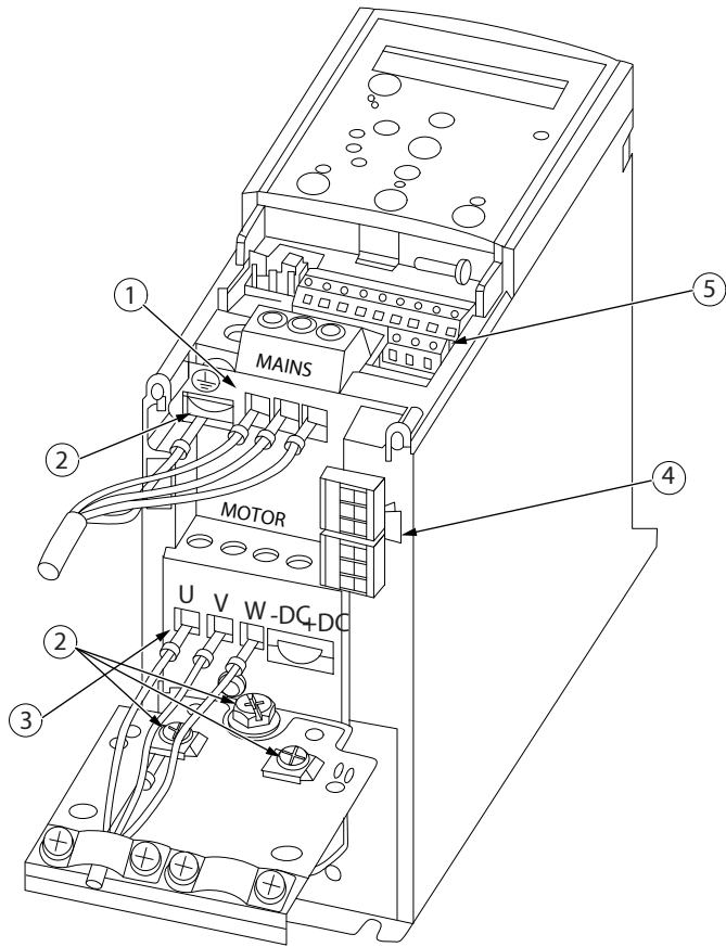
图 56: 机箱规格 H1-H5 IP20, 380-480 V, 0.37-22 kW (0.5-30 hp)
