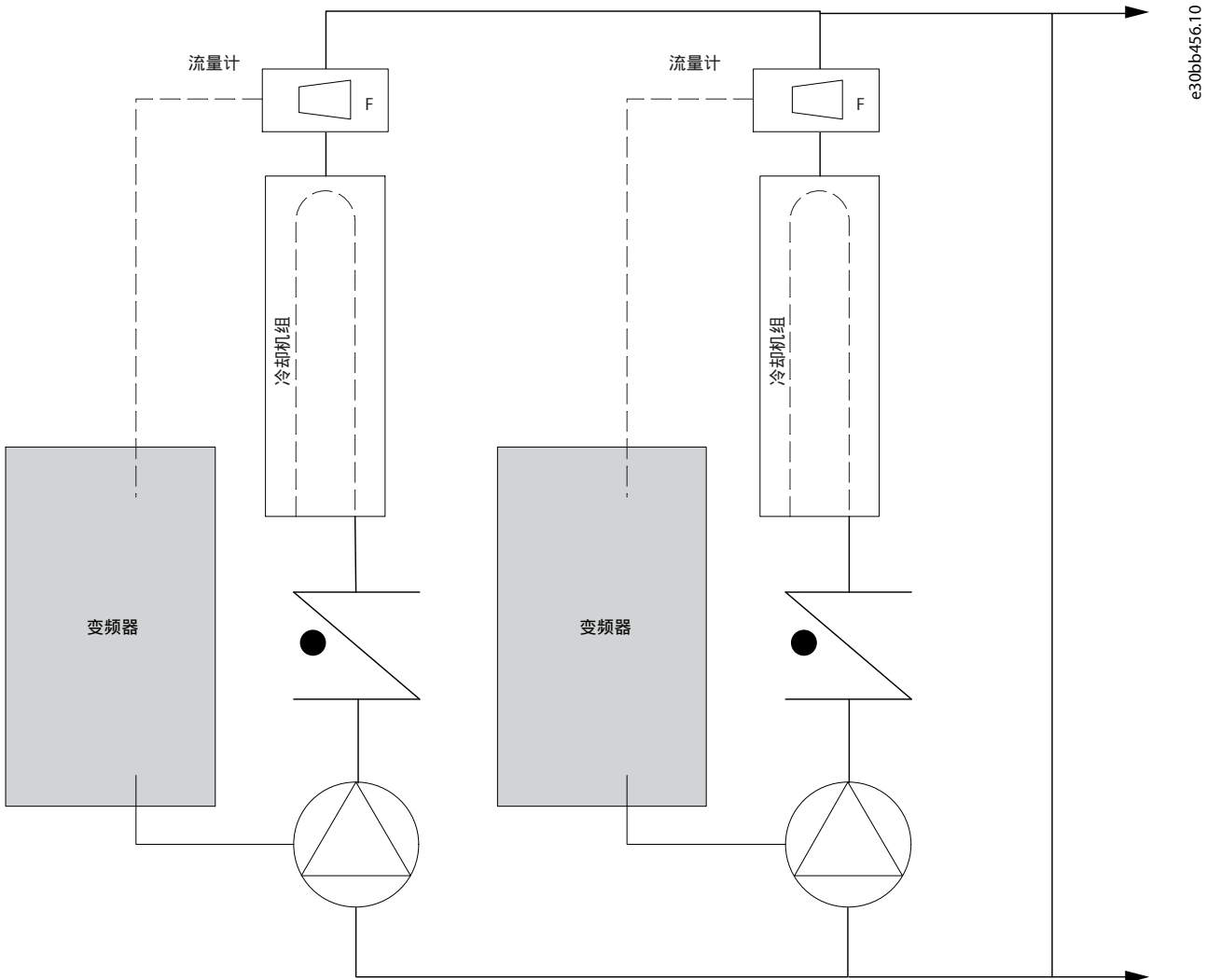
图 15: 主泵
