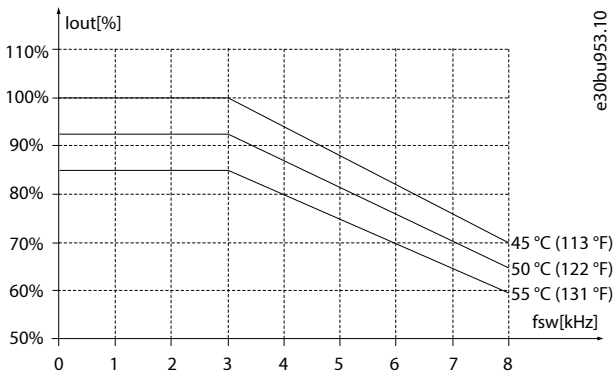
图 52: 110-315 kW (150-450 hp), 400 V, 机箱规格 H13-H14, IP20, 开关模式 60 AVM
