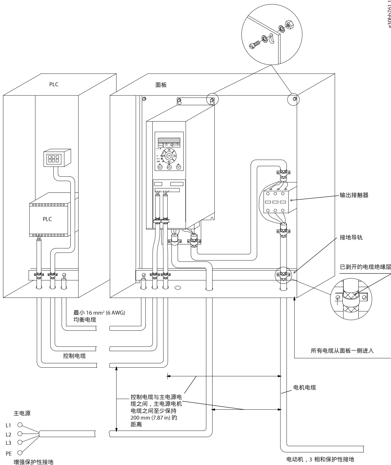
图 55: 符合 EMC 规范的电气安装
