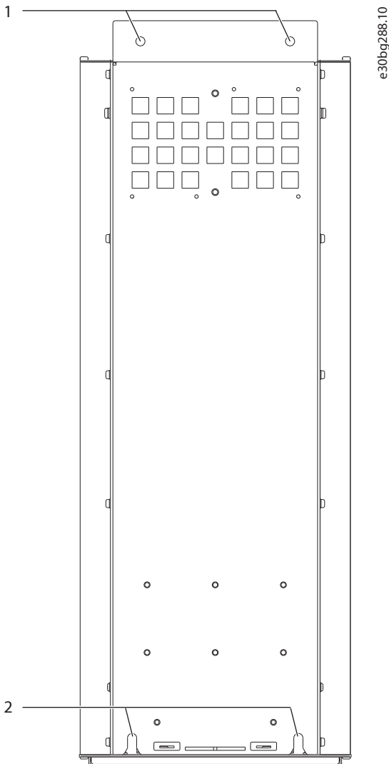
图 42: 变频器壁装孔
