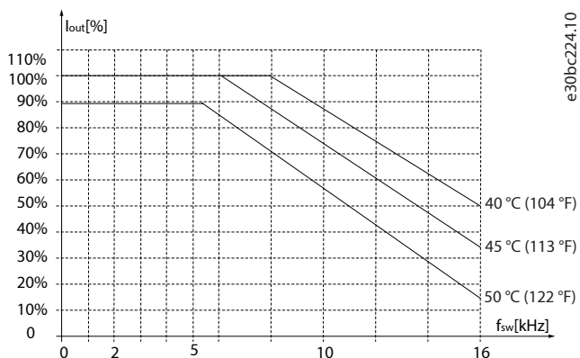
图 47: 11-15 kW (15-20 hp), 400 V, 机箱规格 H4, IP20
