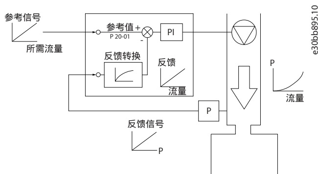
图 20: 反馈信号转换
