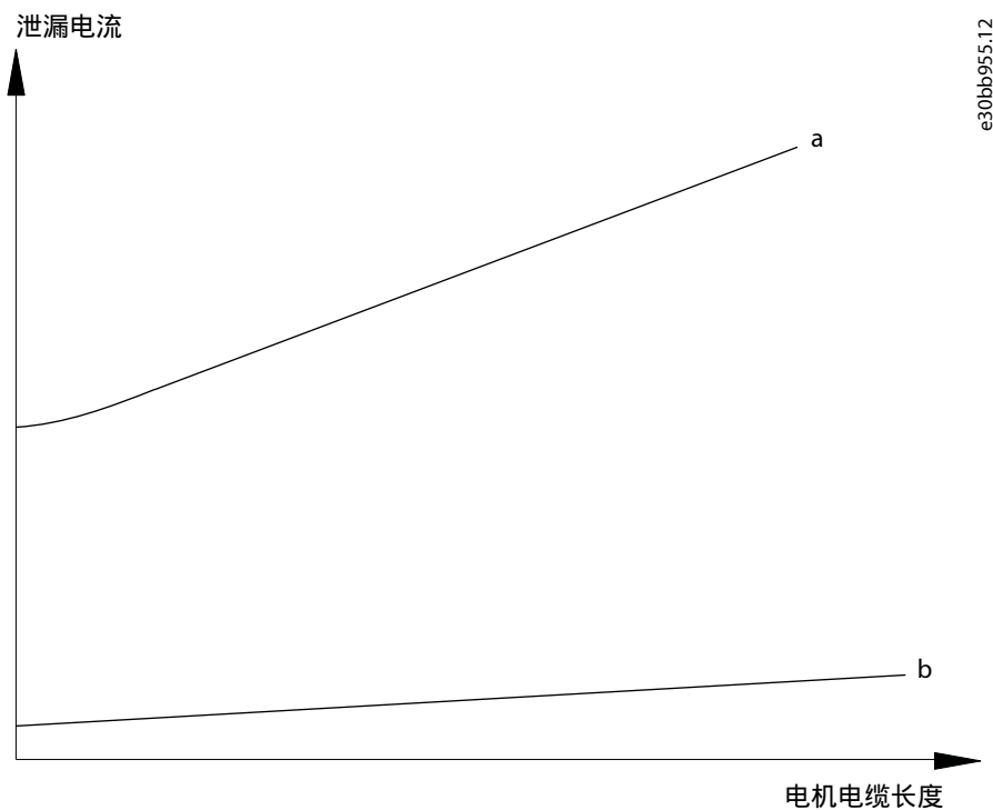
图 27: 电缆长度和功率规格对泄漏电流的影响，功率规格 a > 功率规格 b
