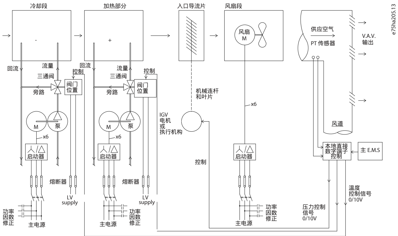
图 9: 无变频器的传统风扇系统
