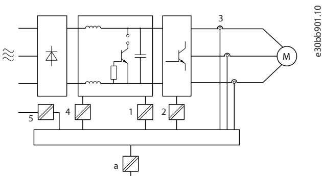
图 25: 电气隔离 30-90 kW (40-120 hp)
