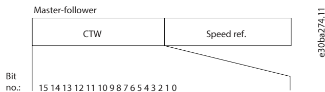
图 84: 与 FC 协议对应的控制字
