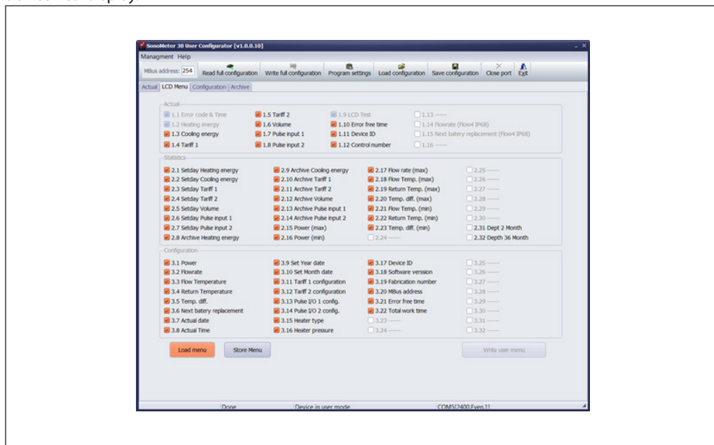
Fig. 5.8 LCD Menu
