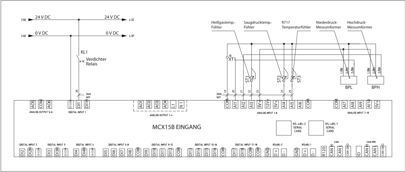
Abb. 19 Regler MCX15B Eingänge
