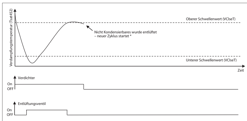
Abb. 3 – Entlüftungsvorgang – Niedrige R452A-Verdampfungstemperatur während des PDT erkannt: Schwellenwerte sind konfigurierbar * Wird eine niedrige Verdampfertemperatur erkannt (unterhalb des unteren Schwellenwertes), wird der Entlüftungsvorgang sofort wiederholt
