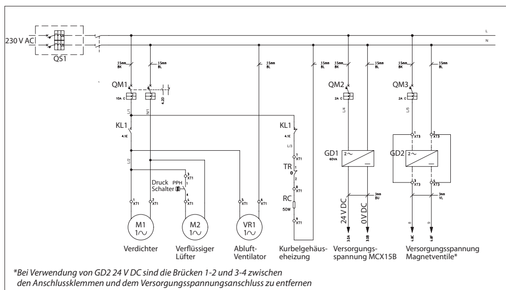
Abb. 17 Versorgungsspannung
