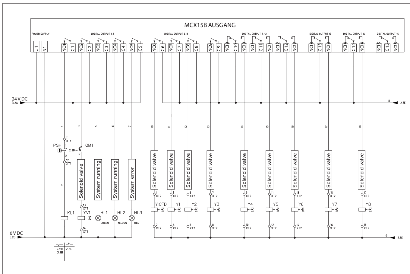
Abb. 18 Regler MCX15B Ein- und Ausgänge
