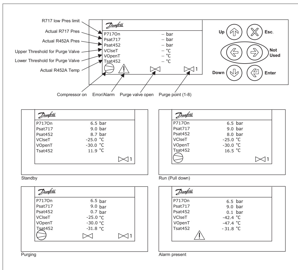
Abb 21 – Standard-Hauptfenster. Betriebs(Start)-Modus (nur Beispiele)
