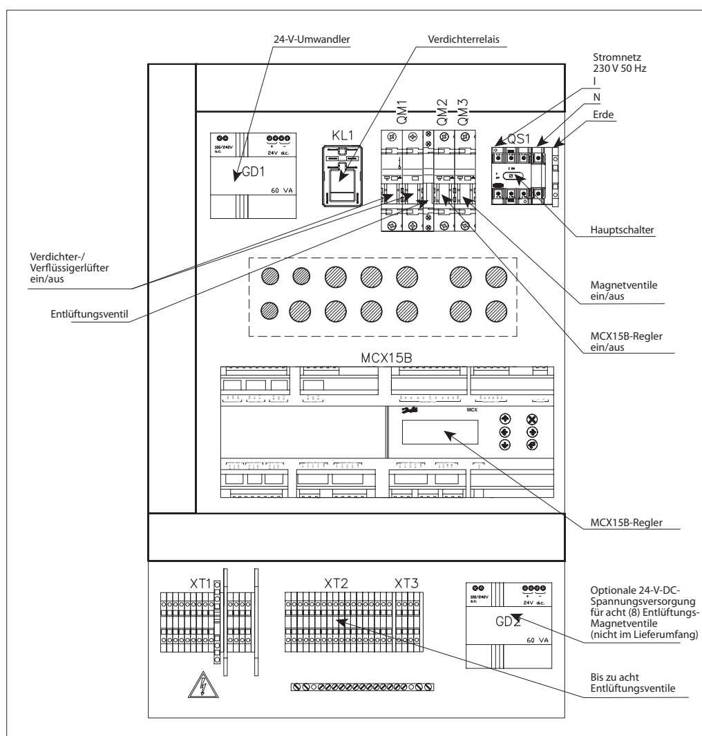
Abb. 16 Regelbox intern
