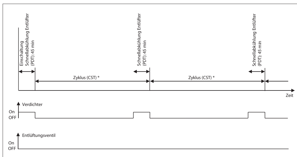
Abb. 2 – Einschalten und Betriebszyklus, wenn keine NC-Gase anwesend sind: CST (Verdichterstartzeit) und PDT (Schnellabkühlzeit) sind konfigurierbar * Zyklus (CST) = 24 Stunden/N (Anzahl Entlüftungspunkte)
