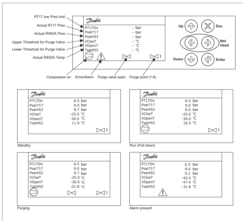
图 21 – 默认主窗口。运行（启动）模式。（仅供参考）
