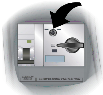
Rys 17. Do przeprowadzenia kalibracji należy użyć śruby regulacyjnej znajdującej się z przodu ochrony przeciążeniowej silnika.
