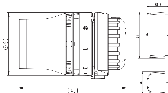
Danfoss Redia® RA z czujnikiem wyniesionym
