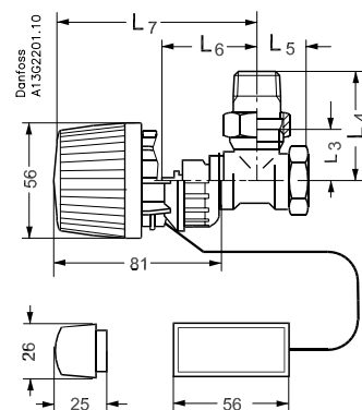
Sarkoszelep RA 2992 érzékelővel
