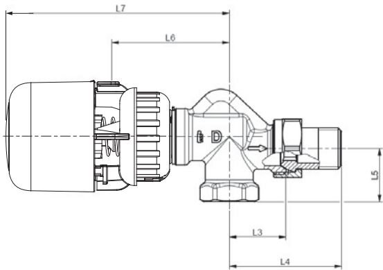
Осьовий клапан RA-DV з термостатичним елементом Aero
