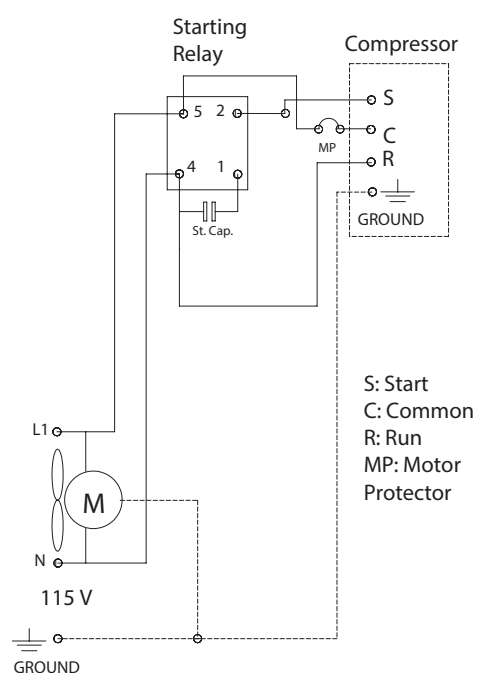
Wiring Diagram 119-3983
