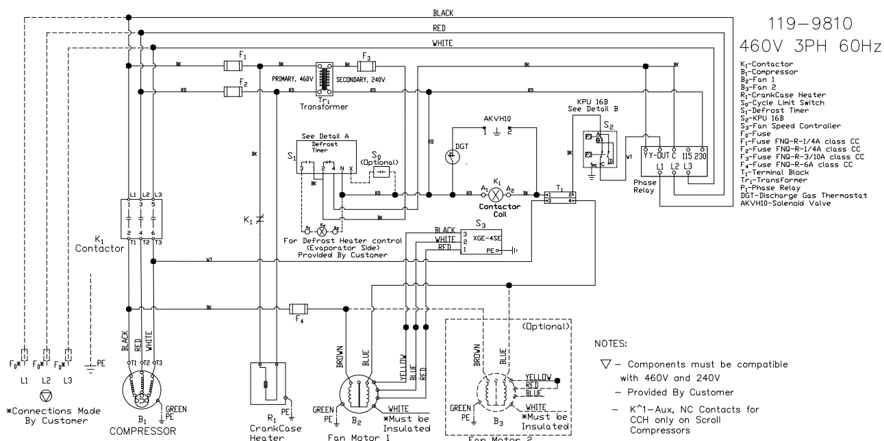
Wiring Diagram 119-9810
