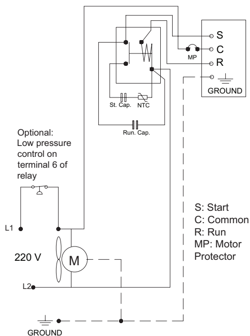
Wiring Diagram 119-9263
