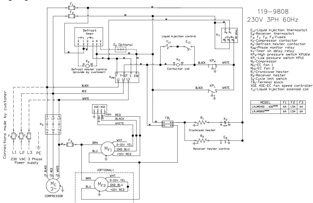
Wiring Diagram 119-9808
