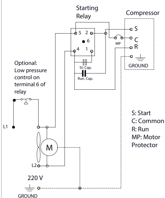
Wiring Diagram 119-3990
