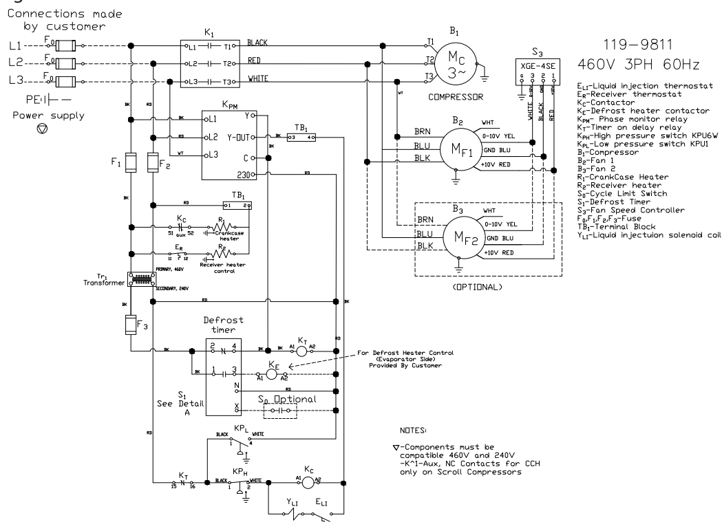
Wiring Diagram 119-9811
