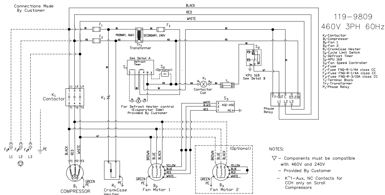
Wiring Diagram 119-9809
