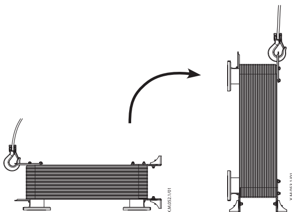
Fig. 2 Lifting / Fig. 2 Løft / Abb. 2 Heben / Fig. 2 Levage / Fig. 2 Elevación / Fig. 2 Sollevamento / Fig. 2 Lyftning / Fig. 2 Hysen / Kuva 2 Nostaminen / 2 pav. Kėlimas / 2. att. Pacelšana / Joonis 2 Tõstmine / Obr. 2 Zdvíhanie / Slika 2 Dviganje / Sl. 2 Podizanje / 图 2 起吊 / Фуз. 2 Повдигане / Slika 2 Podizanje / Fig. 2 Ridicare / 2. ábra: Emelés / Obr. 2 Zvedání / Rys. 2 Podnoszenie / Puc. 2 Подъем
