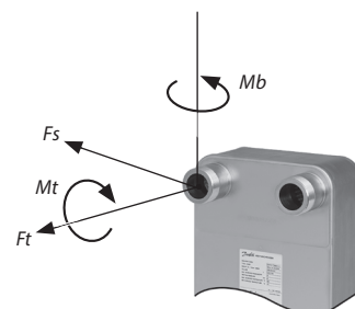
Fig. 3 Torque force / Fig. 3 Drejningsmoment / Abb. 3 Drehmoment / Fig. 3 Force de couple / Fig. 3 Esfuerzo de torsión / Fig. 3 Forza coppia / Fig. 3 Vridmoment / Fig. 3 Torsiekracht / Kuva 3 Vääntävä voima / 3 pav. Sukimo momento jėga / 3. att. Griezes momenta spēks / Joonis 3 Pöördemomendi tugevus / Obr. 3 Sila krútiaceho momentu / Slika 3 Navorna sila / Sl. 3 Sila okretnog momenta / 图 3 扭力 / Фуз. 3 Въртящ момент / Slika 3 Sila obrtnog momenta / Fig. 3 Forța de cuplu / 3. ábra: Azonosító címke / Obr. 3 Kroutivá sila / Rys. 3 Siła momentu obrotowego / Puc. 3 Напряжения, действующие на патрубки
