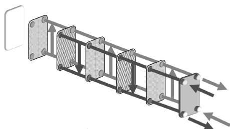
Fig. 4 1-pass / Fig. 4 1-slag / Abb. 4 1-Kreis / Fig. 4 Une passe / Fig. 4 1-paso / Fig. 4 1-passaggio / Fig. 4 1-slags / Fig. 4 1-pass / Kuva 4 1-vetoinen / Fig. 4 1-os pakopos / 4. att. 1 pakāpes / Joonis 4 1-astmeline / Obr. 4 1-prechodový / Slika 4 1-prehod / Sl. 4 Jednoproložni / 图 4 单流程 / Фуз. 4 1-ходов / Slika 4 1-proložni / Fig. 4 1 trecere / 4. ábra: 1 járatú / Obr. 4 1 okruh / Rys. 4 1-stopniowy / Puc. 4 1-ходовая схема
