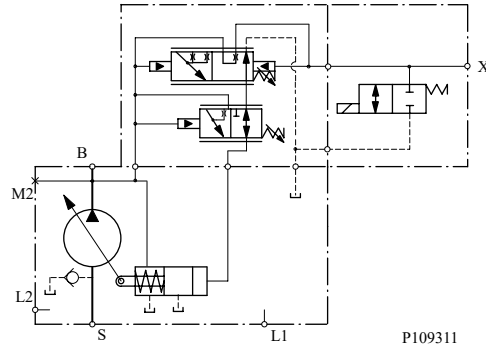
回路図
