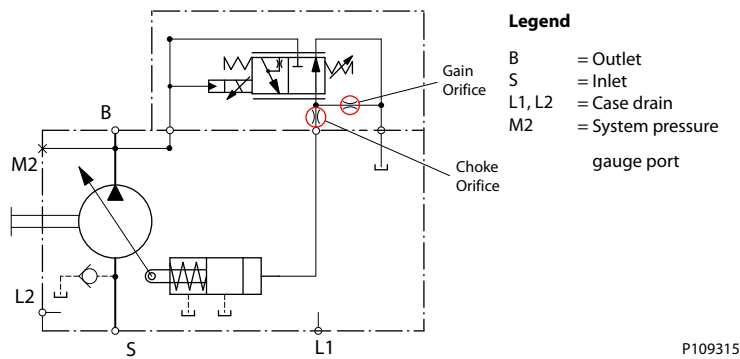
FDC コントロール内蔵のS45 ポンプの回路図
