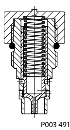
断面図
