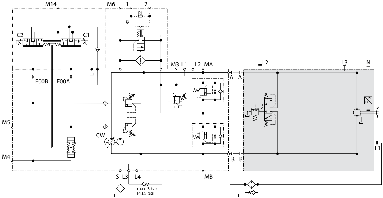
H1 ポンプおよびH1F モータのシステム回路図
