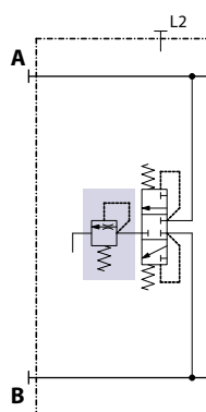
回路図
