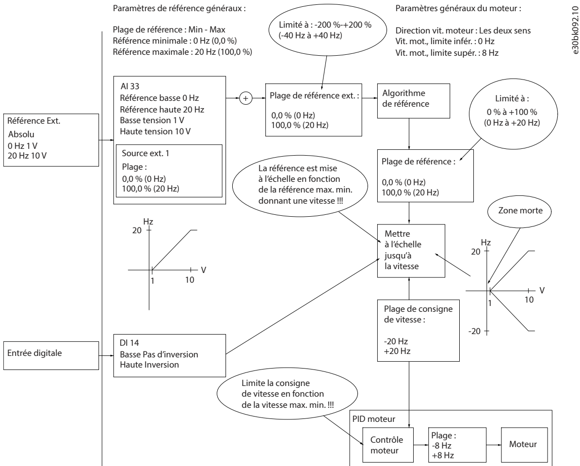
Illustration 49: Verrouillage de l'entrée de référence avec des limites comprises entre Min et Max
