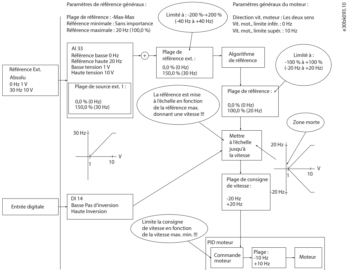
Illustration 50: Verrouillage de l'entrée de référence avec des limites en dehors de -Max à +Max
