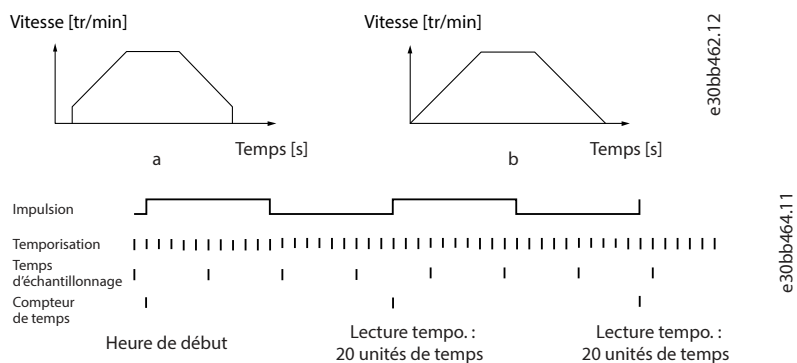
Illustration 85: Durée entre les flancs d'impulsion
