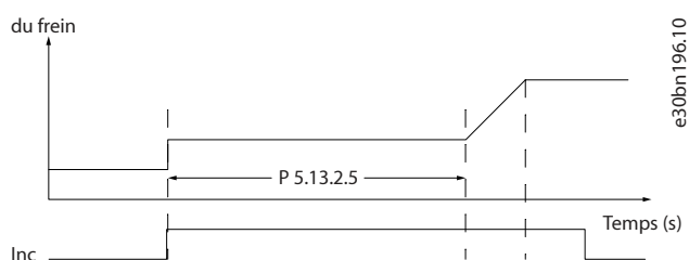
Illustration 80: Augmenter la référence réelle
