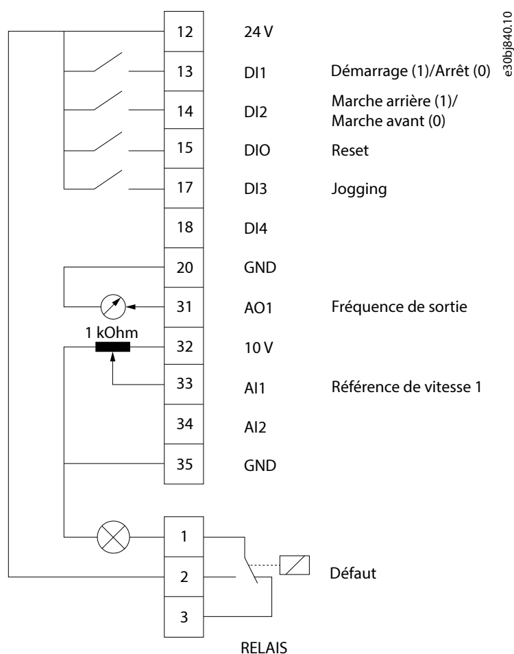
Illustration 37: Connexions par défaut
