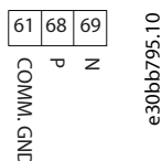
Illustration 52: Raccordement du réseau
