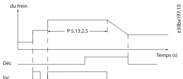
Illustration 81: Augmenter/diminuer la référence réelle
