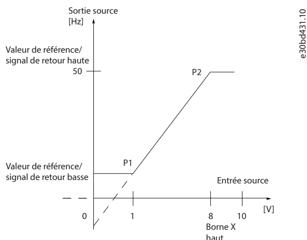
Illustration 47: Valeurs limites minimum et maximum
