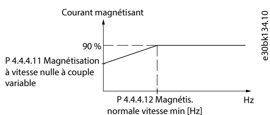
Illustration 73: Magnétisation du moteur
