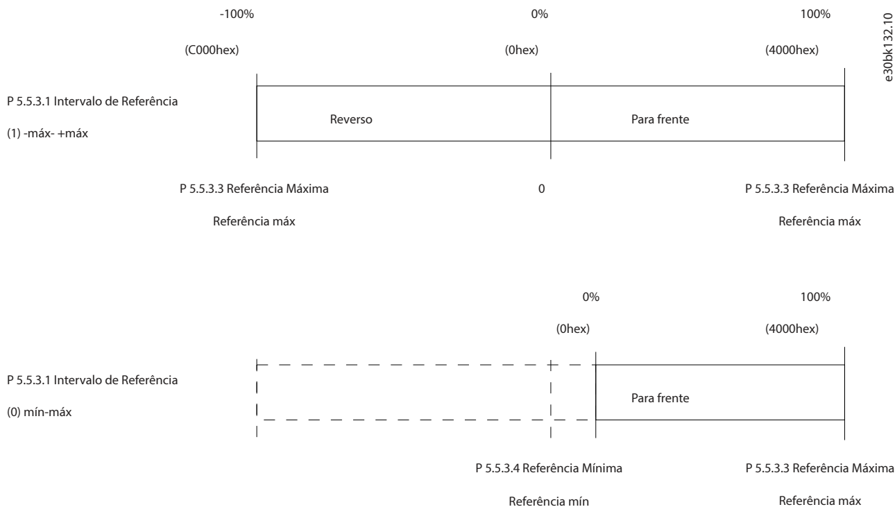
Figura 68: Referência e MAV
