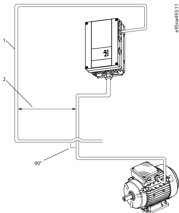
Figura 54: Distância mínima entre cabos de comunicação e potência
