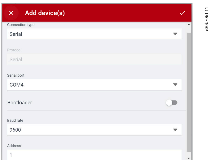
Figura 20: Conexão serial
