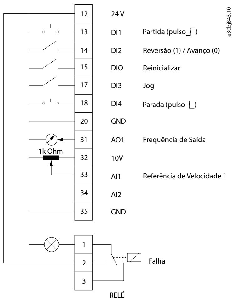
Figura 40: Conexões padrão
