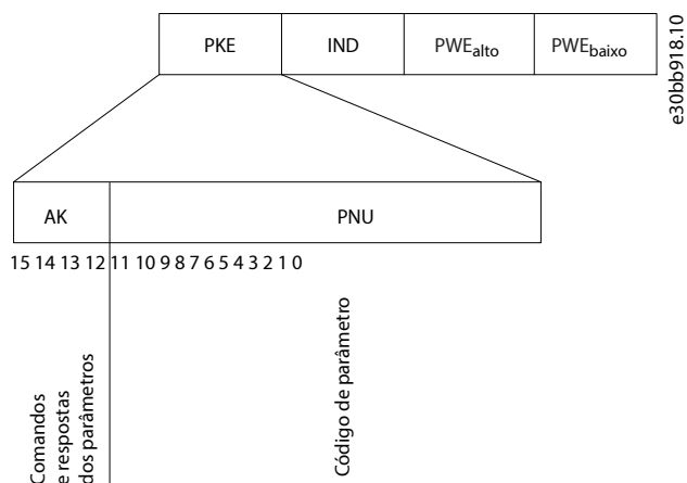
Figura 60: Campo PKE
