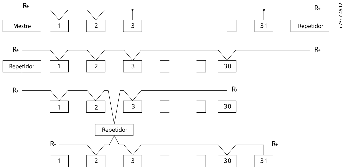
Figura 51: Interface RS-485
