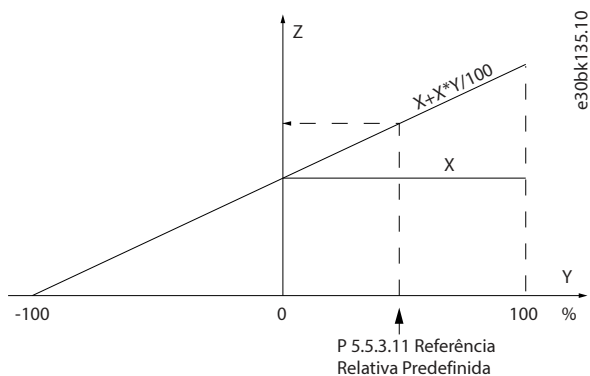
Figura 78: Referência real
