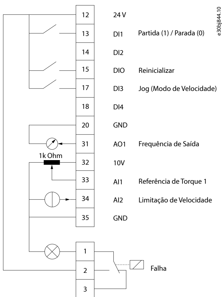
Figura 42: Conexões padrão
