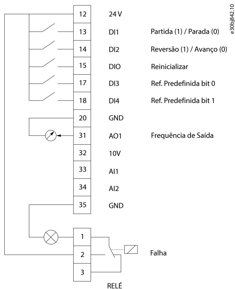
Figura 39: Conexões padrão
