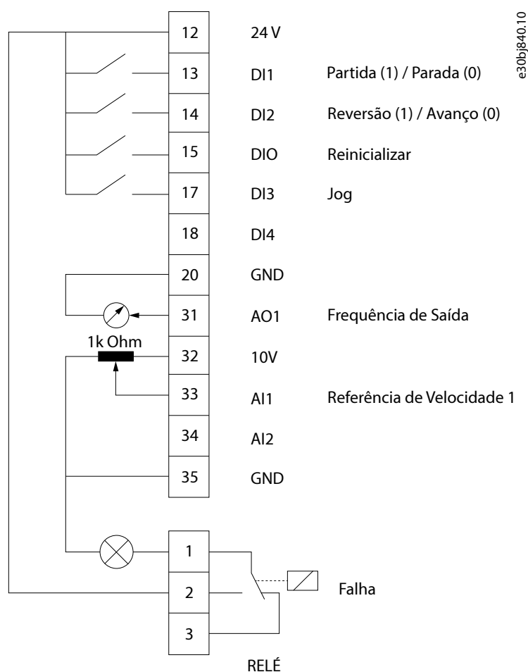
Figura 37: Conexões padrão
