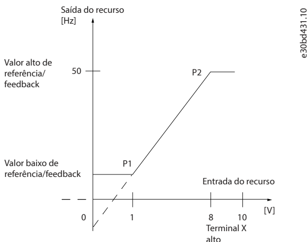
Figura 47: Pontos finais mínimo e máximo
