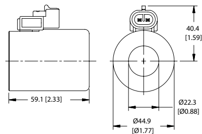
DN DIN 43650
