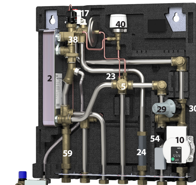
MSS 1, 2, 3 avec circulation
