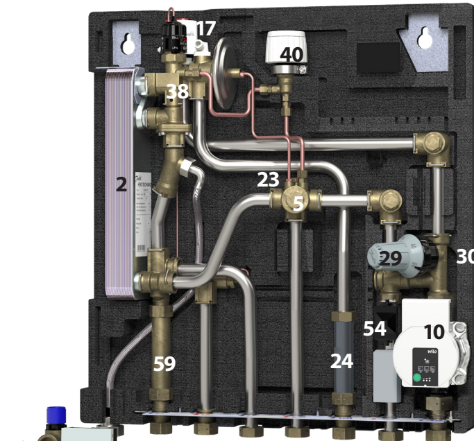
MSS 1, 2, 3 cu recirculare
