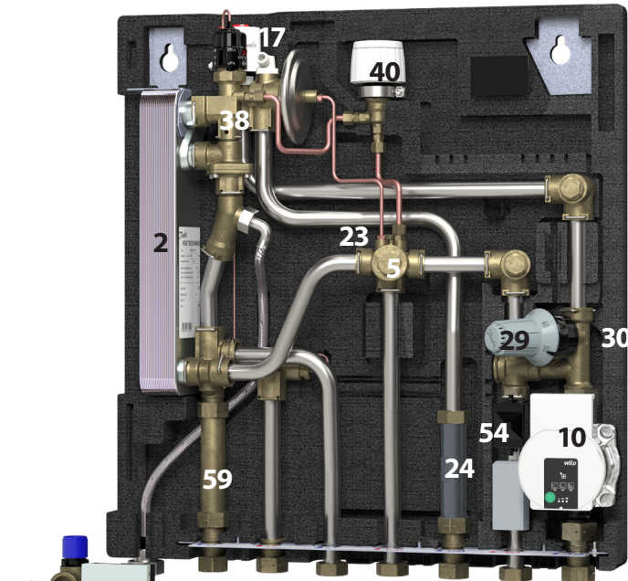
MSS 1, 2, 3 mit Zirkulation
