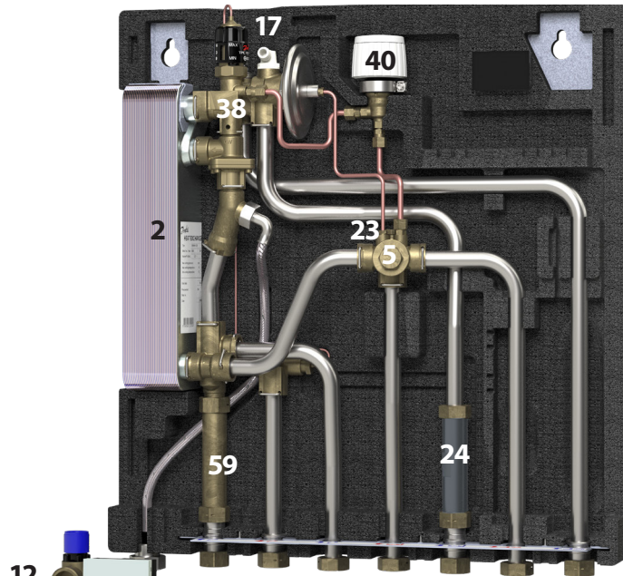
FSS1, 2, 3 mit Zirkulation
