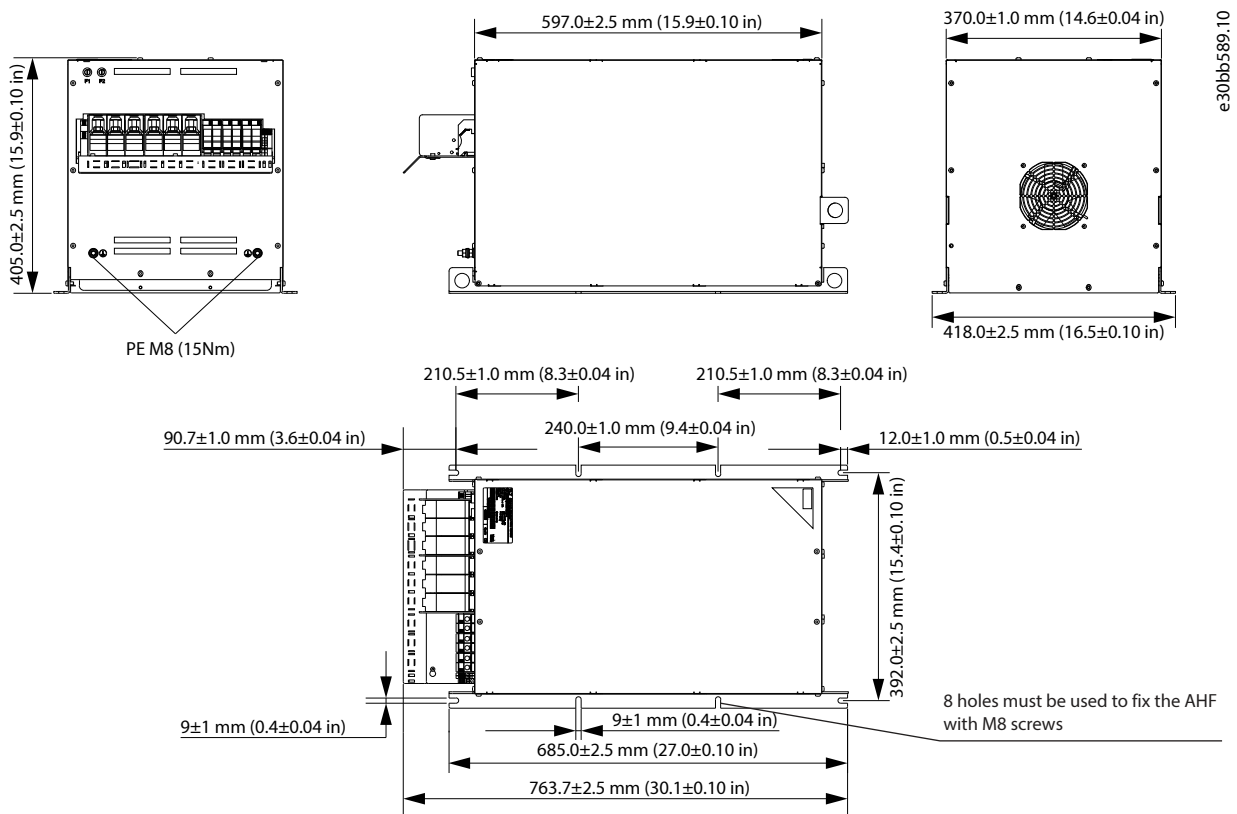
Figure 51: IP20 X6-V3 Internal Fan
