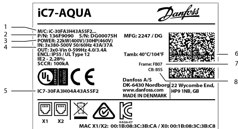
Figura 1: Esempio di etichetta prodotto di un convertitore di frequenza FB07/FK07
