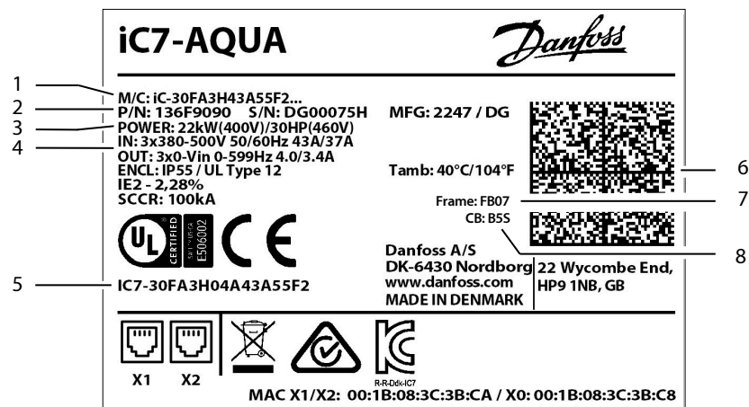
Figura 1: Ejemplo de una etiqueta de producto para FB07/FK07
