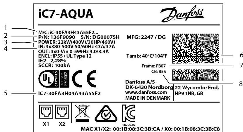
Illustration 1: Exemple d'étiquette de produit FB07/FK07
