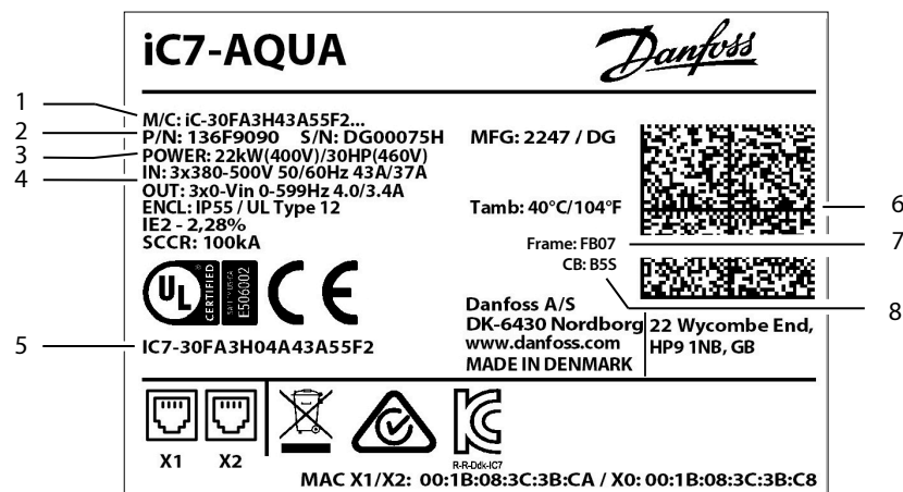
Figura 1: Exemplu de etichetă de produs pentru FB07/FK07
