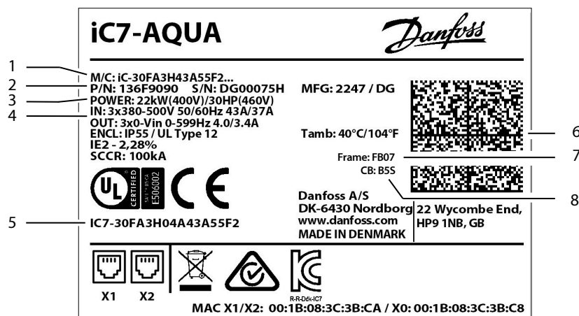
Εικόνα 1: Παράδειγμα ετικέτας προϊόντος FB07/FK07
