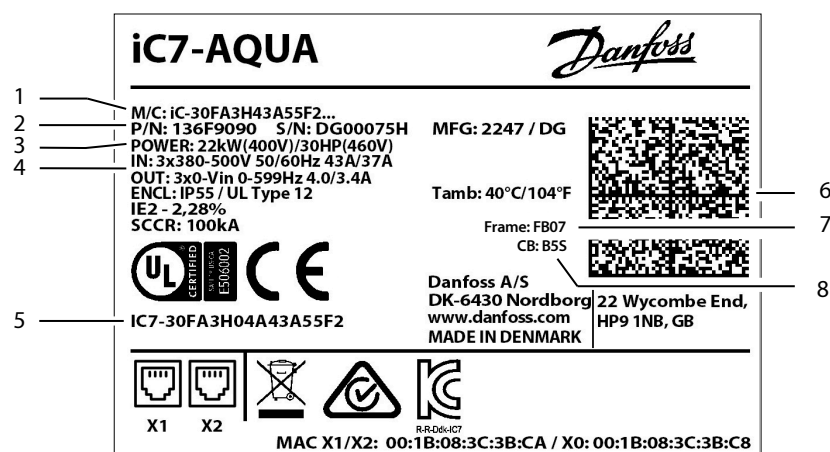
图 1: FB07/FK07 产品标签示例
