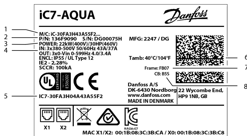
Obrázek 1: Příklad typového štítku FB07/FK07
