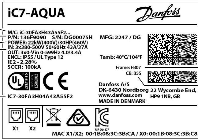
شكل 1: مثال على ملصق المنتج FB07/FK07
