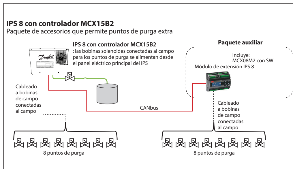
Fig. 10e 8 puntos de purga extra
