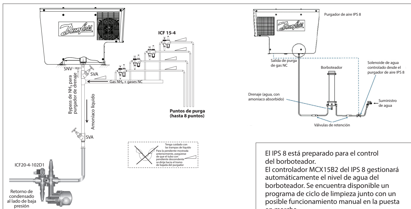
Fig. 10b Purga de varios puntos hasta un máximo de 8 puntos de purga e ICFD como válvula de drenaje
