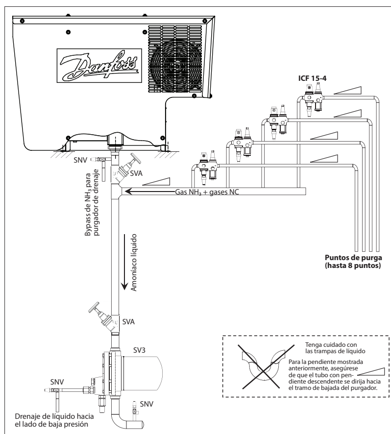
Fig. 10 Purga de varios puntos hasta un máximo de 8 puntos de purga
