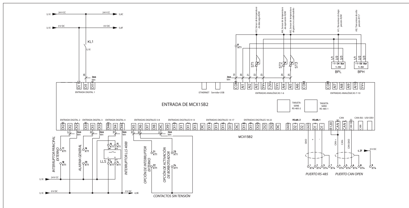
Fig. 19 Entradas del controlador MCX15B2
