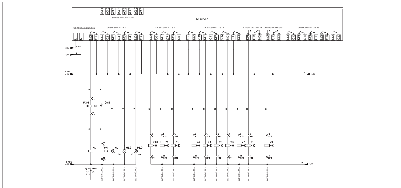
Fig. 17 Fuente de alimentación
