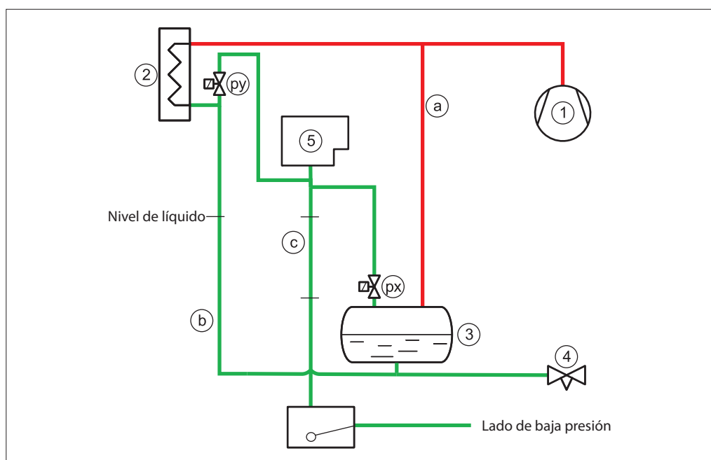
Fig. 7 Conexiones del purgador (px) y (py). El tubo de drenaje (c) debe estar colocado en vertical o con una pendiente descendente
