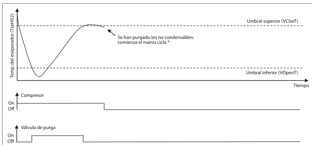
Fig. 3. Procedimiento de purga. Temperatura de evap. baja del R290 detectada durante la PDT: Los umbrales se pueden configurar
