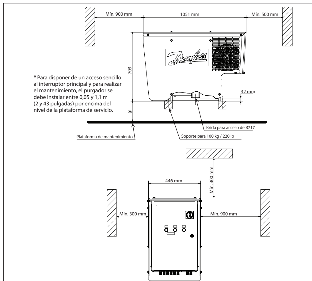
Fig. 12 Dimensiones de la instalación
