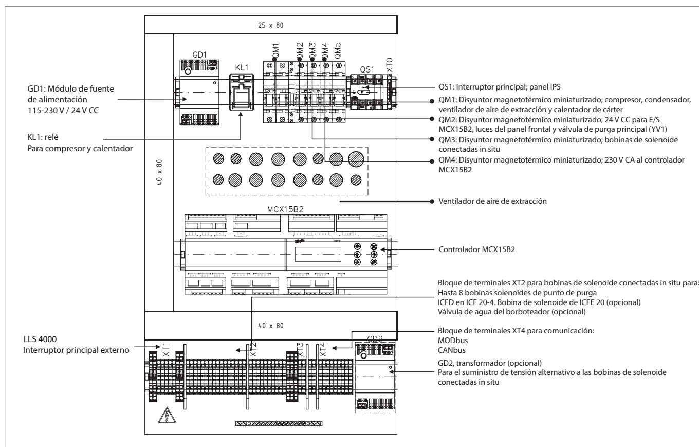
Fig. 16 Caja de control interna
