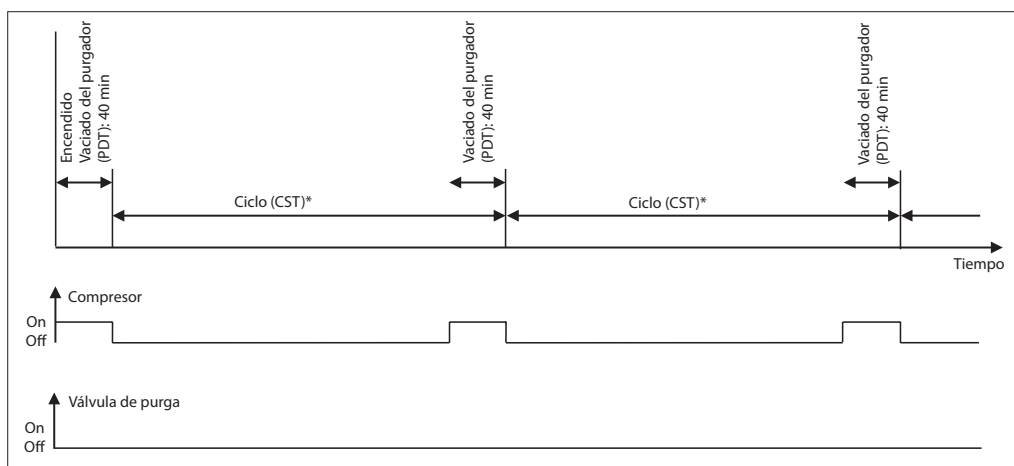
Fig. 2 - Encendido y ciclo sin gases NC presentes: es posible configurar la CST (hora de arranque del compresor) y la PDT (hora de ciclo de vaciado)
