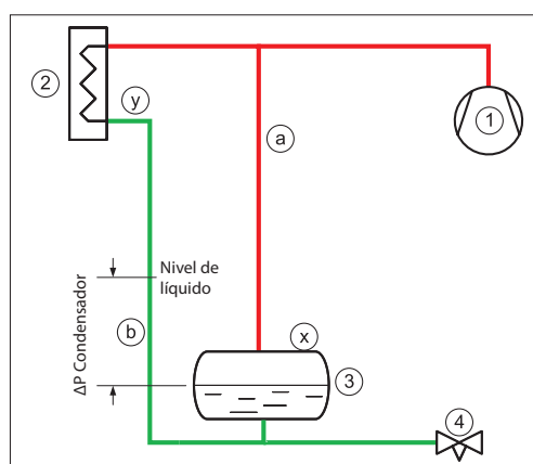
Fig. 4 Nivel de líquido. Recipiente con conexión inferior
