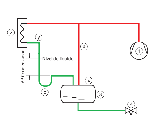
Fig. 5 Nivel de líquido. Recipiente con conexión superior
