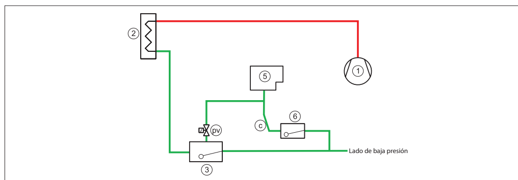
Fig. 8 Conexiones del purgador (pv). El tubo de drenaje (c) debe estar colocado en vertical o con una pendiente descendente
