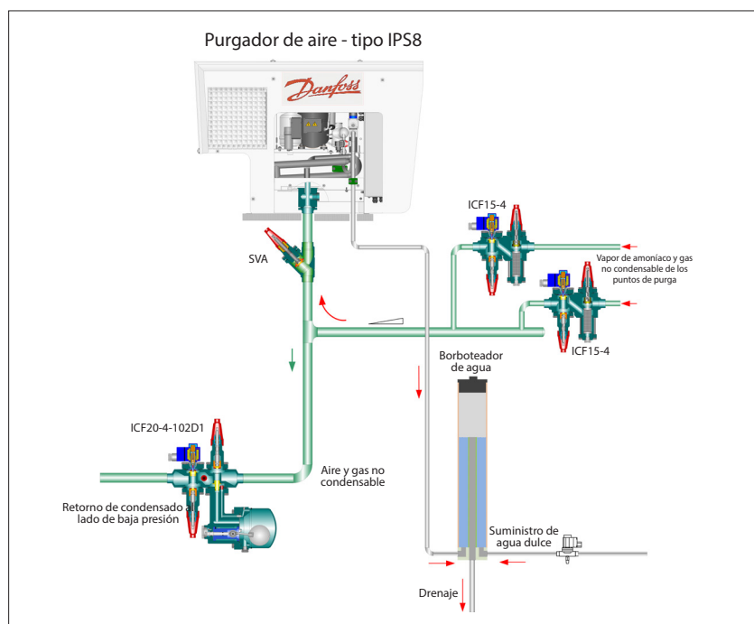
Fig. 10c Purga de varios puntos de hasta un máximo de 8 puntos de purga, ICFD como válvula de drenaje y borboteador
