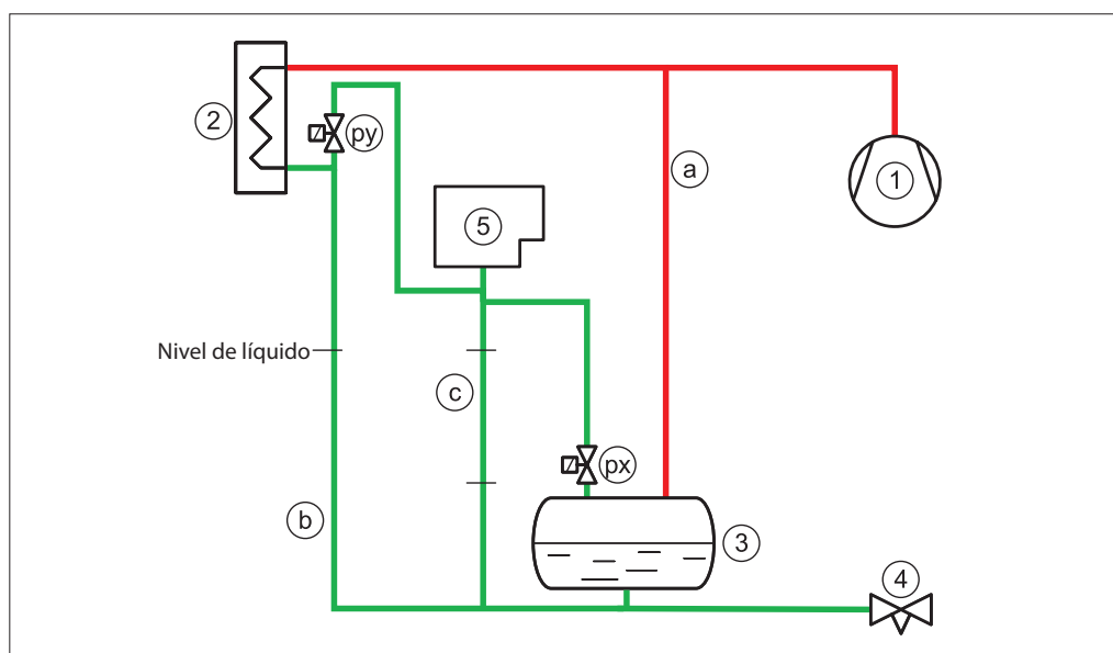
Fig. 6 Conexiones del purgador (px) y (py). El tubo de drenaje (c) debe estar colocado en vertical o con una pendiente descendente
