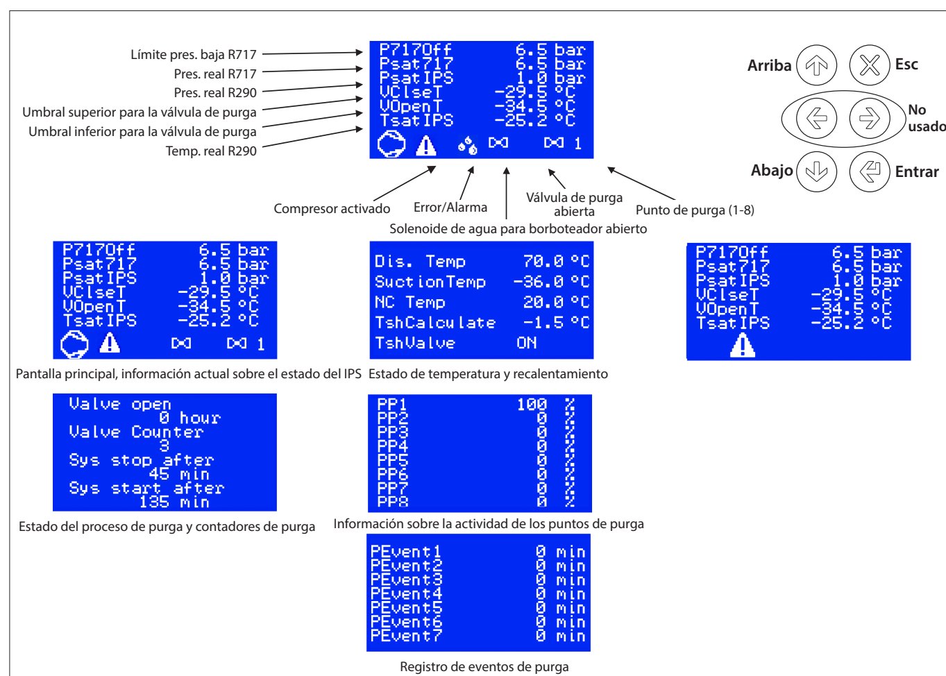
Fig. 21. Ventana principal predeterminada. Modo de funcionamiento (arranque). (Solo ejemplos)
