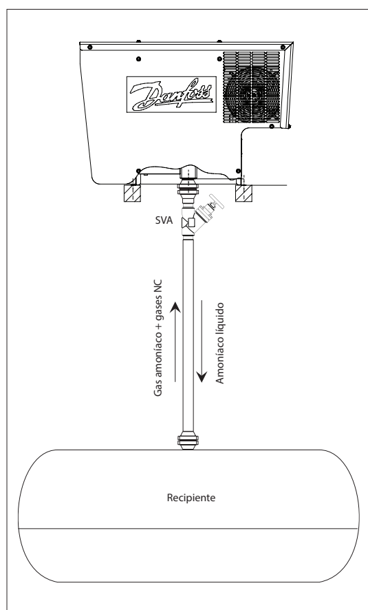
Fig. 9 Purga en un único punto desde el receptor
