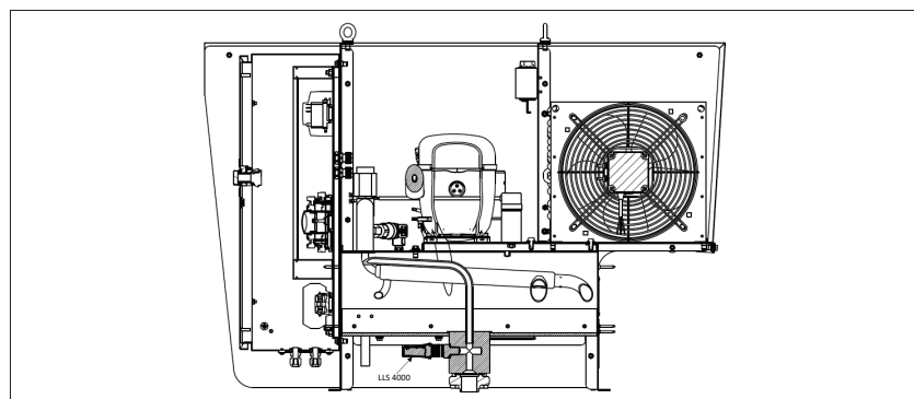
Fig. 10d IPS con LLS 4000 instalado
