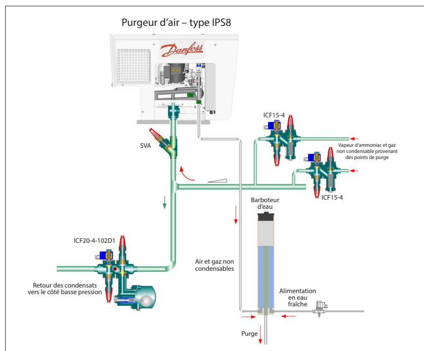
Fig. 10C.1 Activation du barboteur
