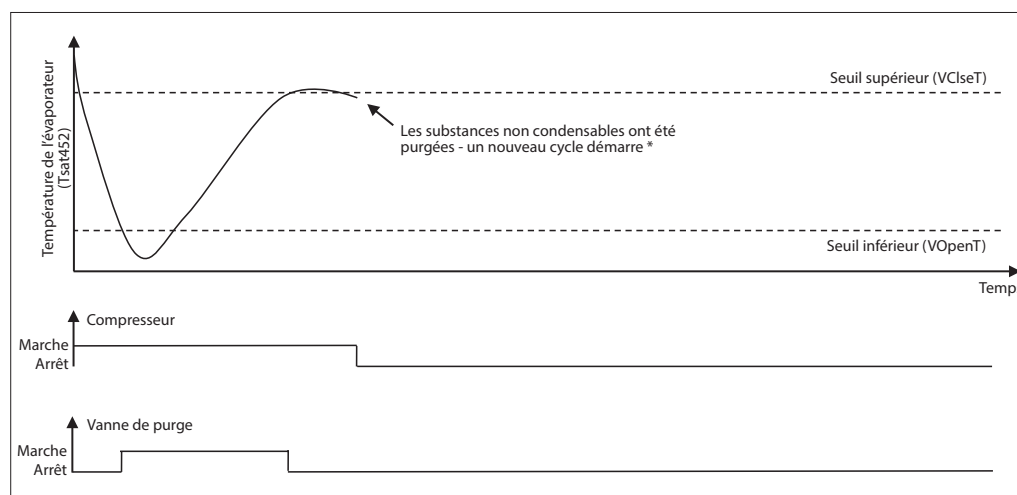
Fig. 3 Procédure de purge - Température d'évaporation R290 basse détectée pendant le PDT : Les seuils peuvent être configurés
