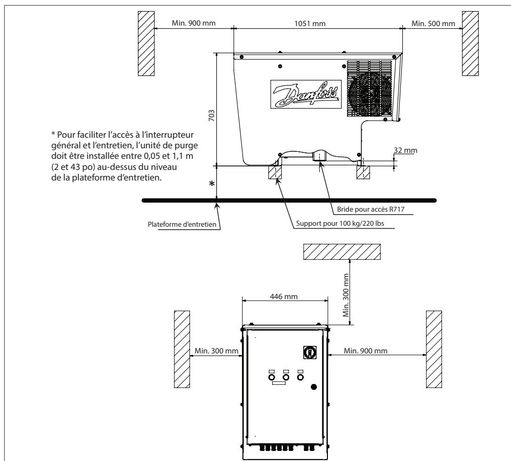
Fig. 12 Dimensions d'installation
