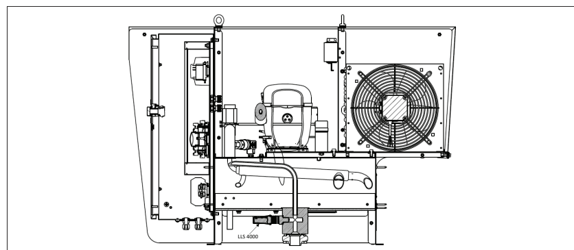
Fig. 10d IPS avec LLS 4000 installé
