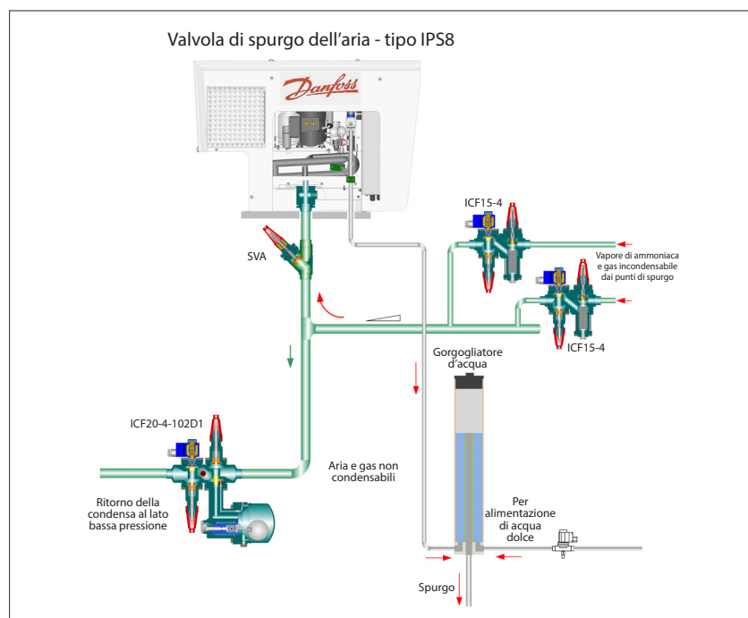
Fig. 10C.1 Attivazione del gorgogliatore
