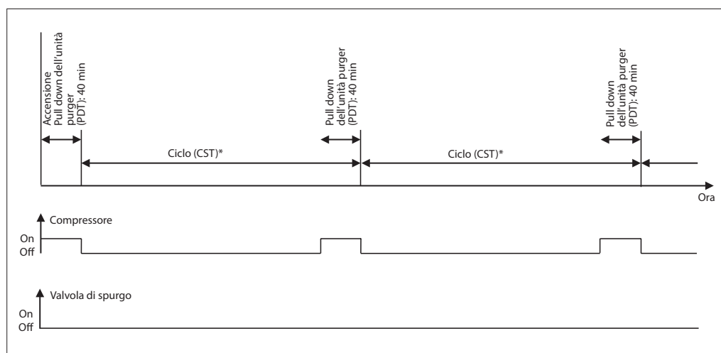
Fig. 2 Accensione e ciclo in assenza di gas N.C.: I valori CST (orario inizio compressore) PDT (orario di pull down) sono configurabili
