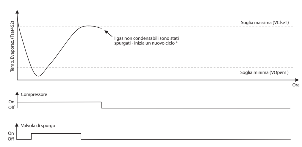
Fig. 3 Procedura di spurgo - Temperatura di evap. di R290 bassa rilevata durante il PDT: Le soglie sono configurabili
