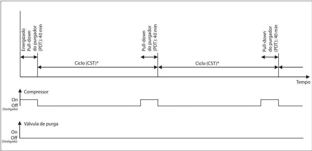
Fig. 2 Energização e ciclo sem a presença de gases não condensáveis: CST (hora de início do compressor) e PDT (hora do pulldown) são configuráveis. * Ciclo (CST) = 24 horas/N (quantidade de pontos de purga)
