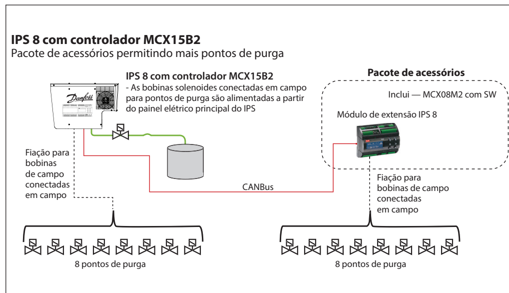
Fig. 10e Mais 8 pontos de purga
