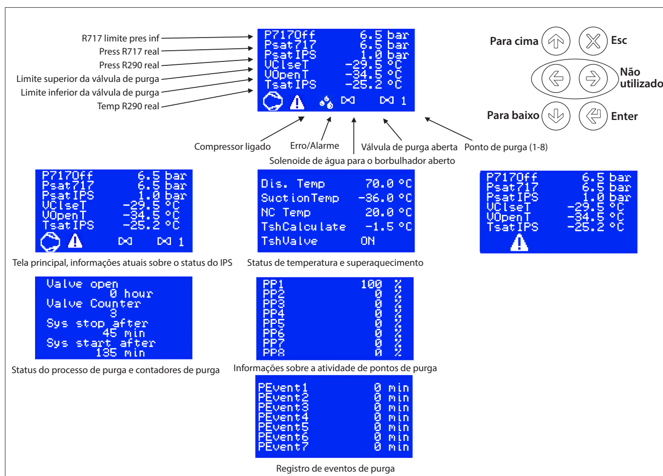
Fig. 21 Janela principal padrão. Modo de operação (inicialização). (Apenas exemplos)
