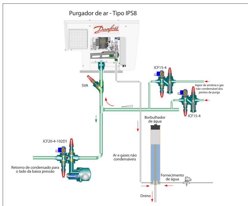
Fig. 10c Purga multipontos de até 8 pontos de purga, ICFD como válvula de drenagem e borbulhador
