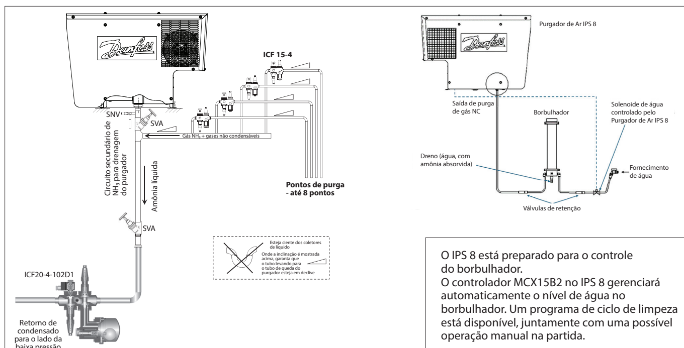
Fig. 10b Purga multipontos de até 8 pontos de purga e ICFD como válvula de drenagem
