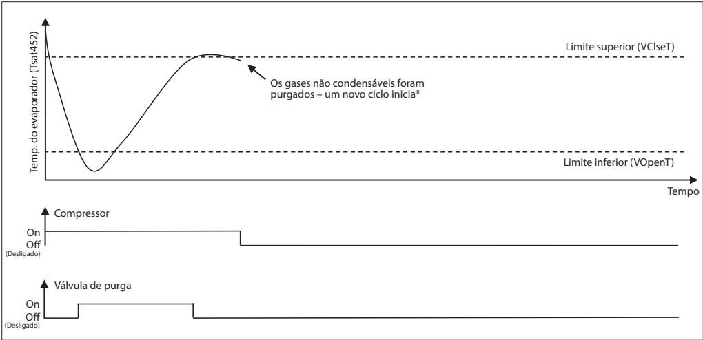
Fig. 3 Procedimento de purga – Baixa temperatura de evap. do R290 detectada durante a PDT: Os limites são configuráveis. * Se uma baixa temperatura do evaporador for detectada (ultrapassando o limite inferior), o procedimento de purga será repetido imediatamente
