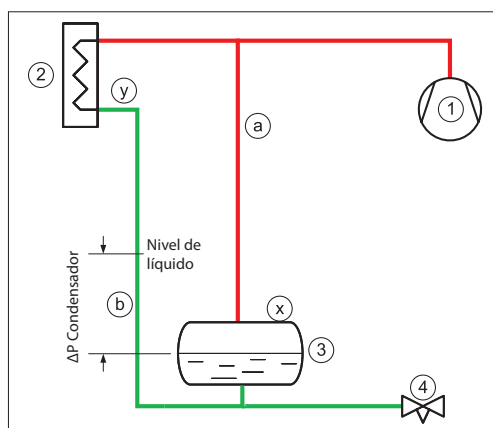
Fig. 4 Nivel de líquido. Recipiente con conexión inferior
