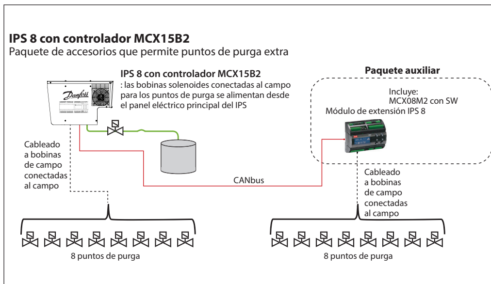
Fig. 10e 8 puntos de purga extra
