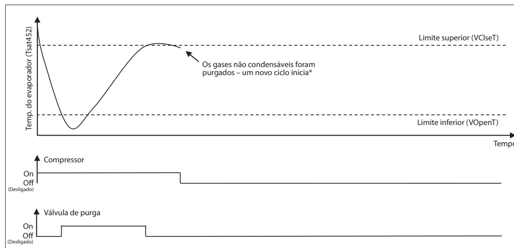
Fig. 3 Procedimento de purga – Baixa temperatura de evap. do R290 detectada durante a PDT: Os limites são configuráveis.
