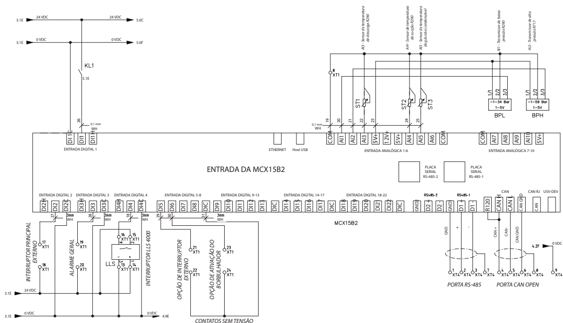
Fig. 19 Entradas do controlador MCX15B2
