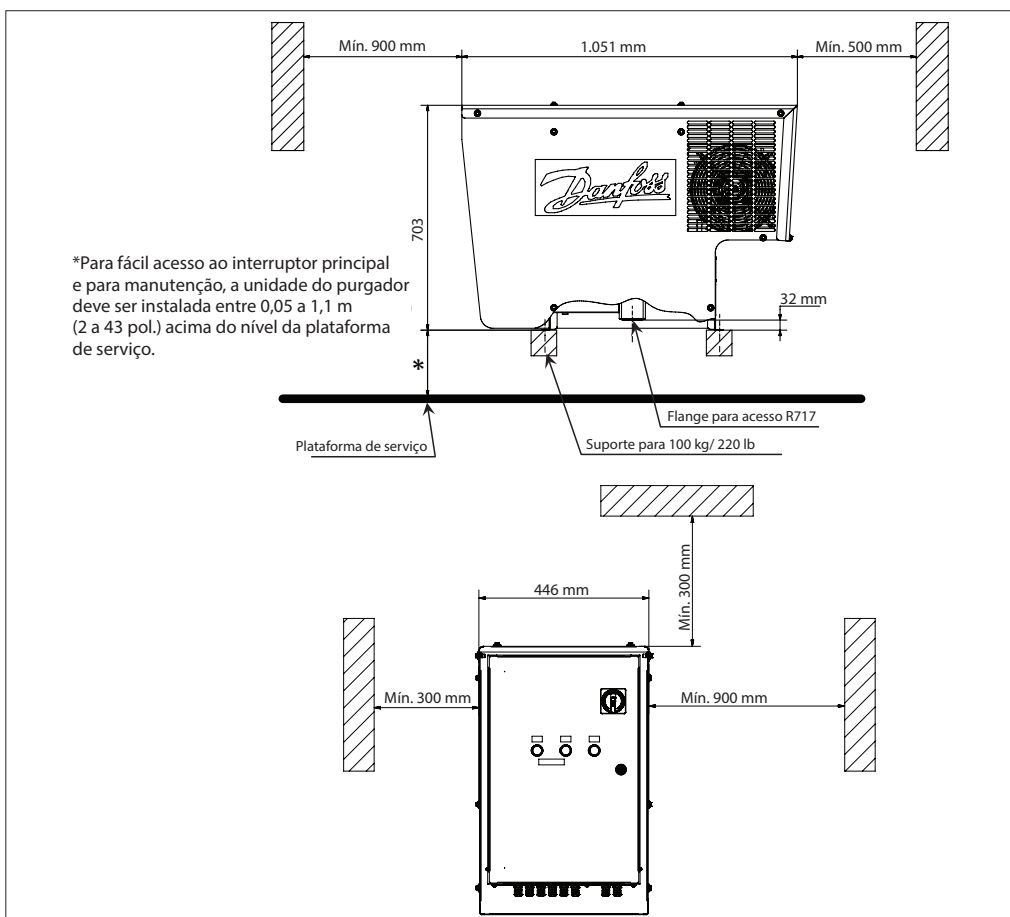
Fig. 12 Dimensões de instalação
