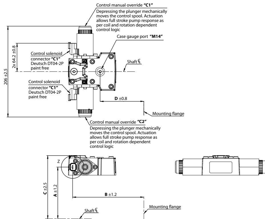
制御ソレノイドコネクタ "C1" & "C2"
