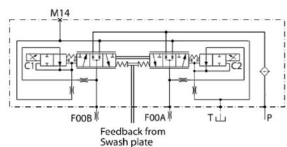
NFPE 回路図
