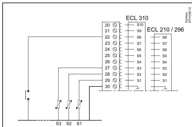
Eksempel: Tilslutning af et overstyringsrelæ
