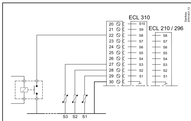
Eksempel: Tilslutning af et overstyringsrelæ
