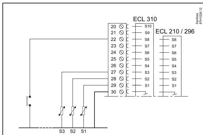
Przykład: Podłączenie przekaźnika sterowania zewnętrznego
