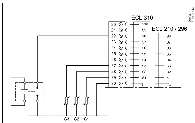
Przykład: Podłączenie przekaźnika sterowania zewnętrznego
