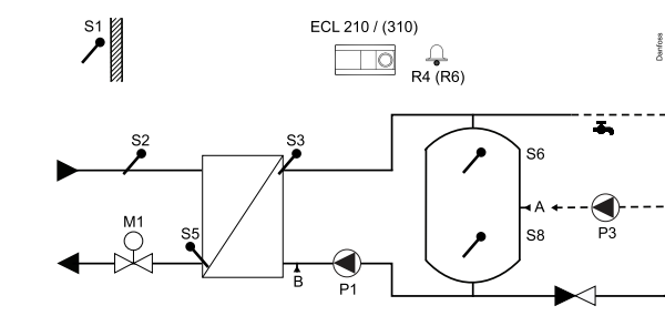
A217.1/A317.1, przykład b:
