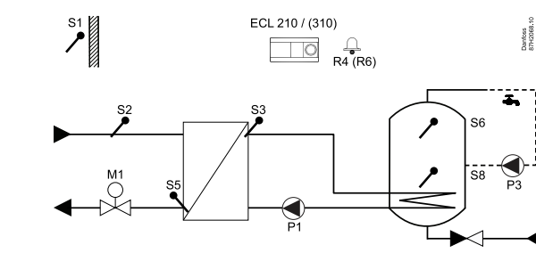
A217.1/A317.1, przykład c:
