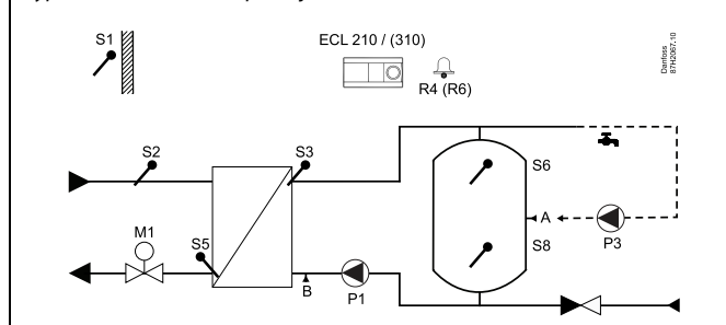
Typowe zastosowanie aplikacji A217.1./A317.1:
