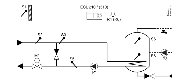
A217.1/A317.1, przykład d:
