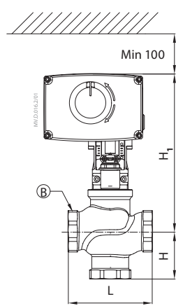
AME 438 SU + VRB 3
