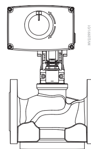
AME 438 SU + VF 3, VL 3 (DN 15-50)
