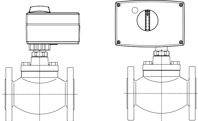
AMV(E) 10, AMV(E) 13 VB2 D_y = 15-20 мм
