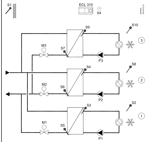
Стандартная схема A390.3:
