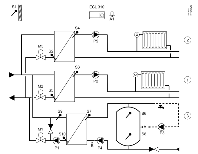
Стандартная схема A390.12: (до 2 контуров отопления, 1 контур ГВС)
