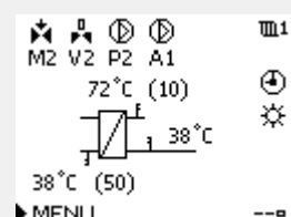
Übersichtsanzeige 4:
