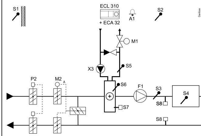
Typische A314.2-Anwendung:
