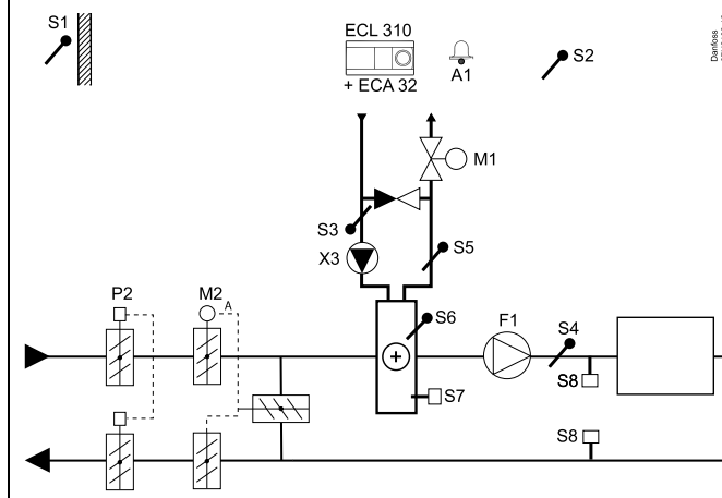
Typische A314.1-Anwendung:
