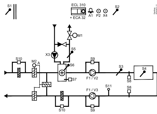
Typische A314.9-Anwendung:
