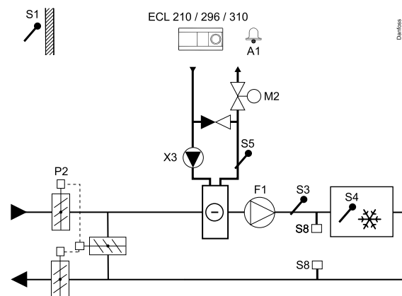
Typische A214.1-Anwendung:
