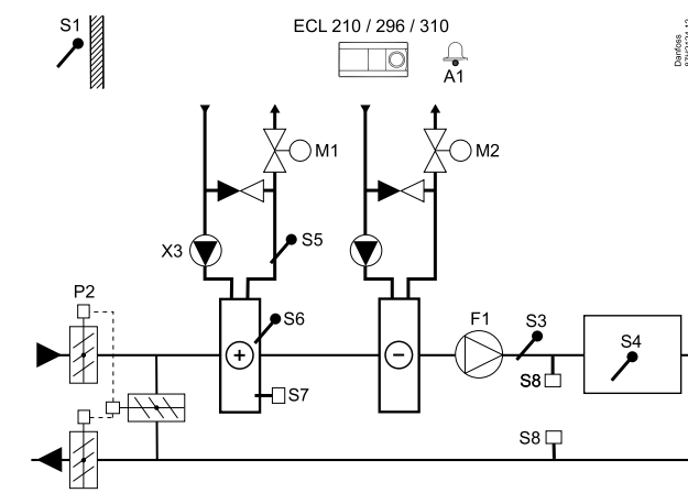
Typische A214.5-Anwendung:
