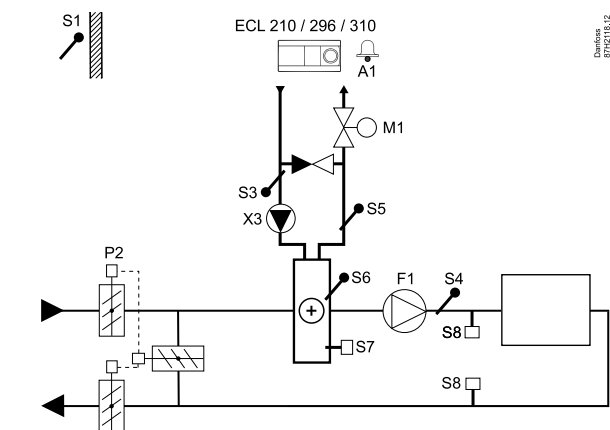
Typische A214.2-Anwendung:
