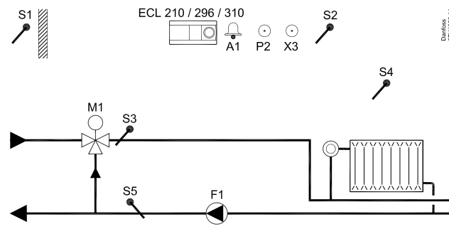
Typische A214.6-Anwendung:
