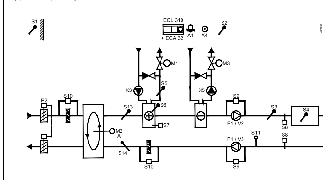
Typowa aplikacja A314.7:
