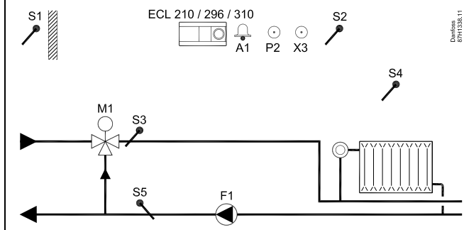
Typowa aplikacja A214.6:
