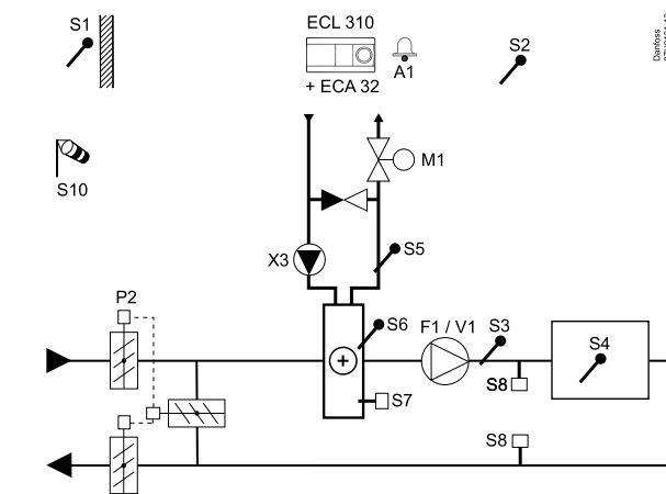
Typowa aplikacja A314.3:
