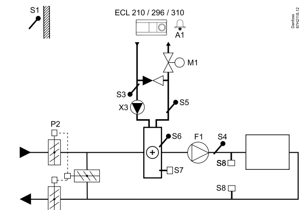
Typowa aplikacja A214.2:
