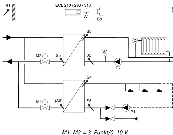
Typische A266.9-Applikation:
