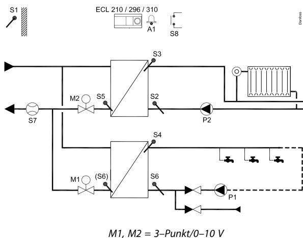
Typische A266.10-Applikation:
