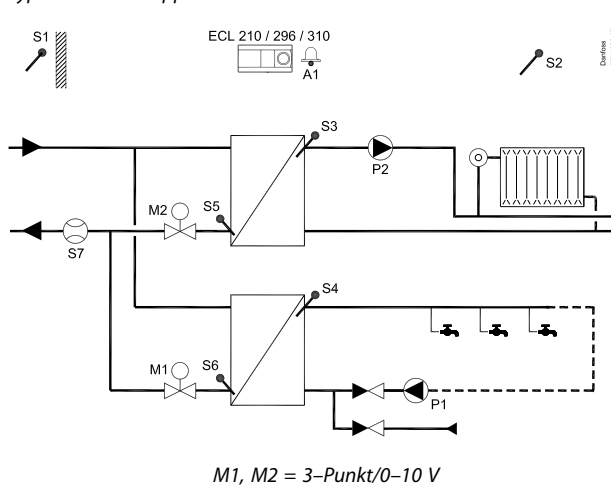
Typische A266.1-Applikation:
