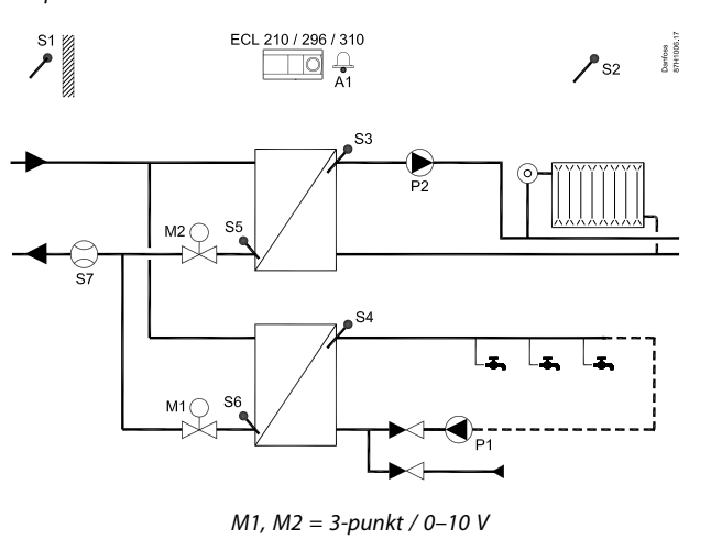
Tüüpiline A266.1 rakendus:
