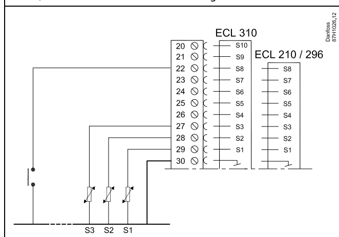
Näide, tühistamislüliti ühendatud sisendiga S8:
