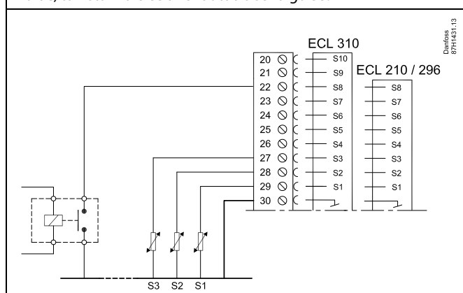
Näide, tühistamisrelee ühendatud sisendiga S8:
