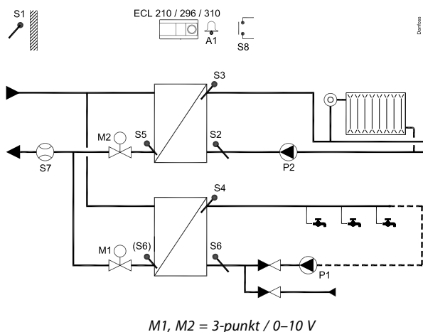
Tüüpiline A266.10 rakendus:
