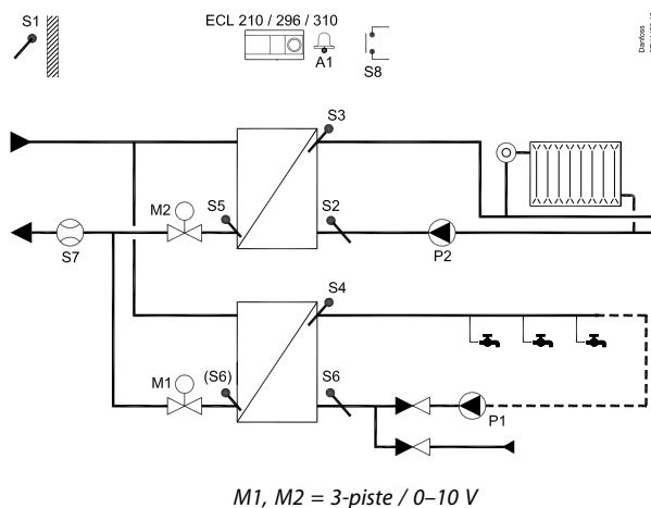
Tyypillinen A266.10-sovellus:
