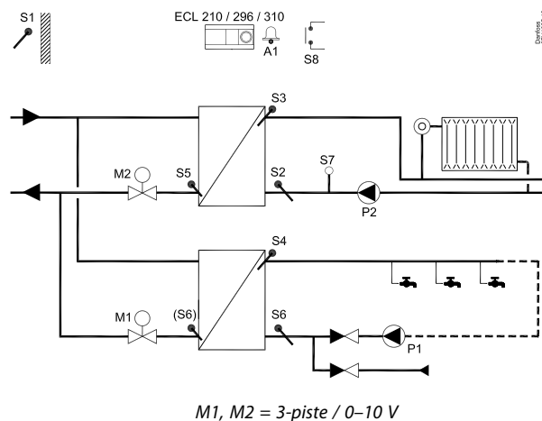
Tyypillinen A266.9-sovellus:
