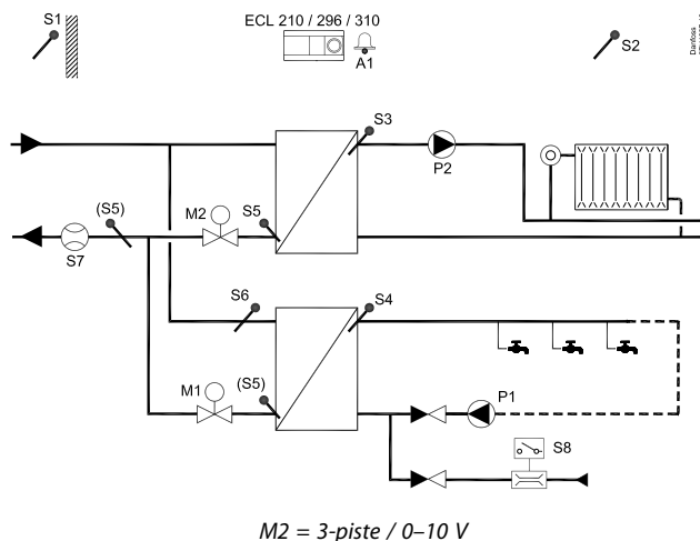
Tyypillinen A266.2-sovellus:
