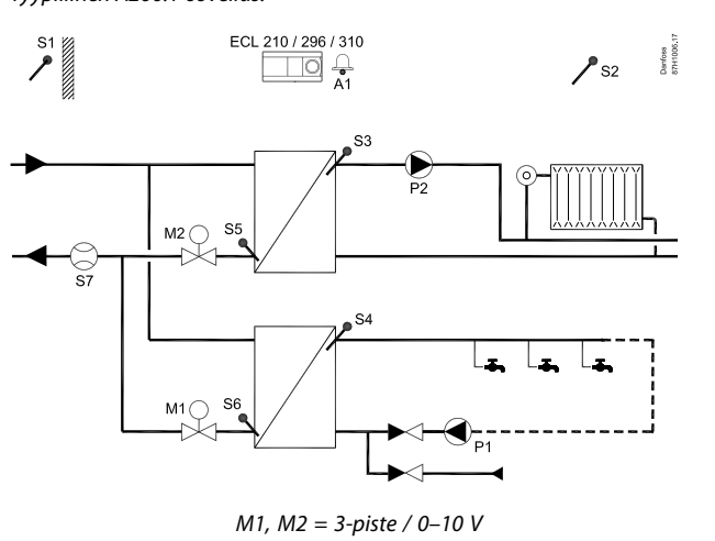
Tyypillinen A266.1-sovellus:
