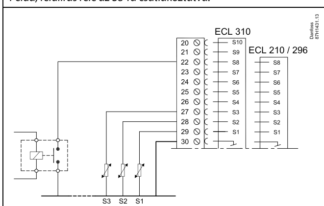
Példa, felülírás relé az S8-ra csatlakoztatva:
