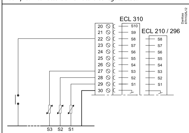
Esempio: interruttore di forzatura collegato a S8:
