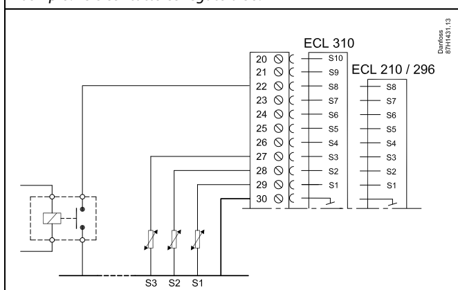
Esempio: relè contatto collegato a S8:
