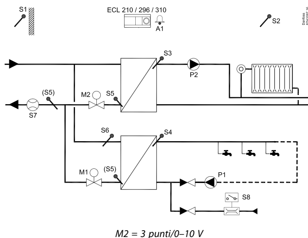
Applicazione A266.2 tipica:
