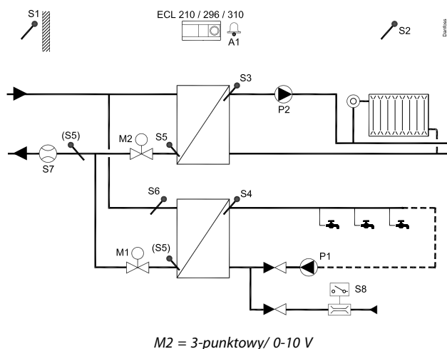
Typowy układ aplikacji A266.2:
