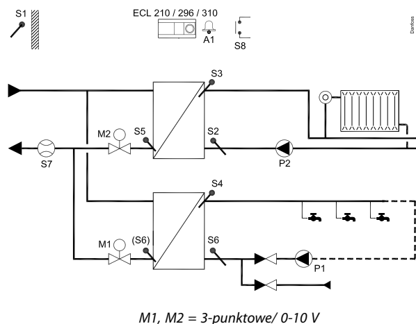
Typowy układ aplikacji A266.10:
