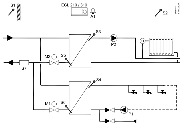
Стандартная схема A266.1:
