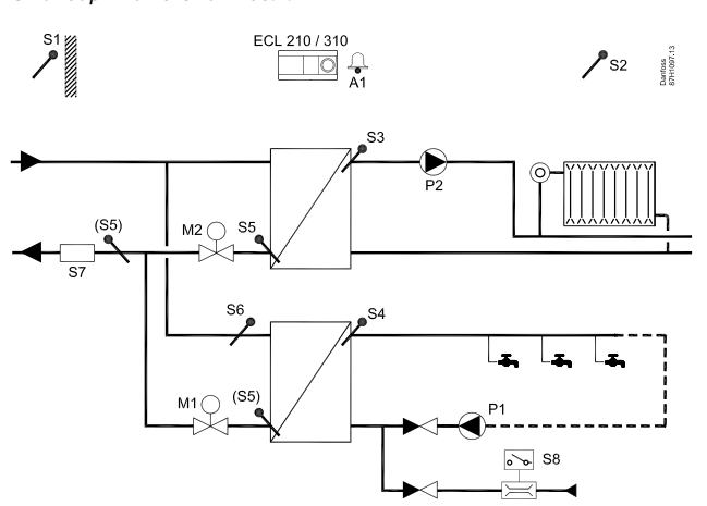
Стандартная схема A266.2:
