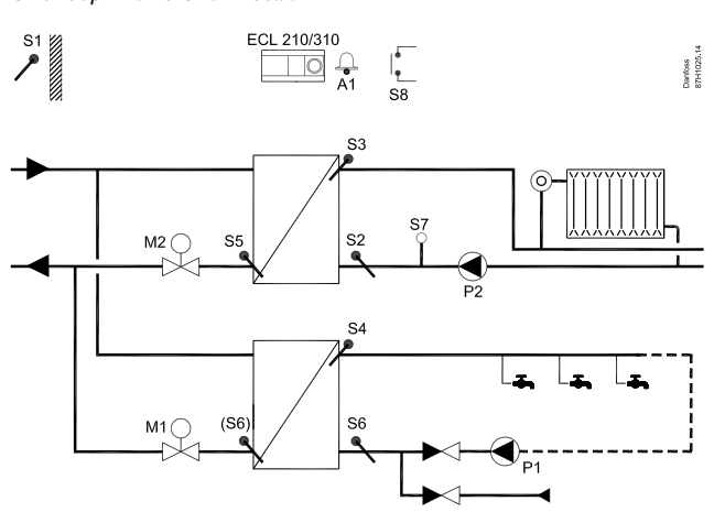
Стандартная схема A266.9:
