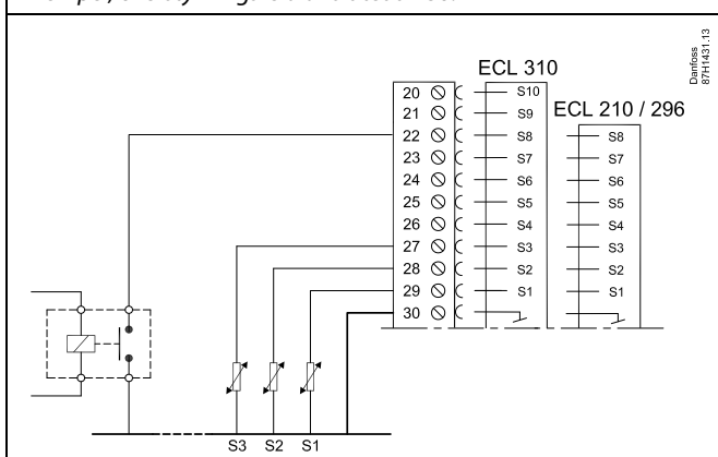
Exempel, överstyrningsrelä anslutet till S8:
