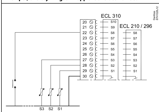
Exempel, överstyrningsomkopplare ansluten till S8:
