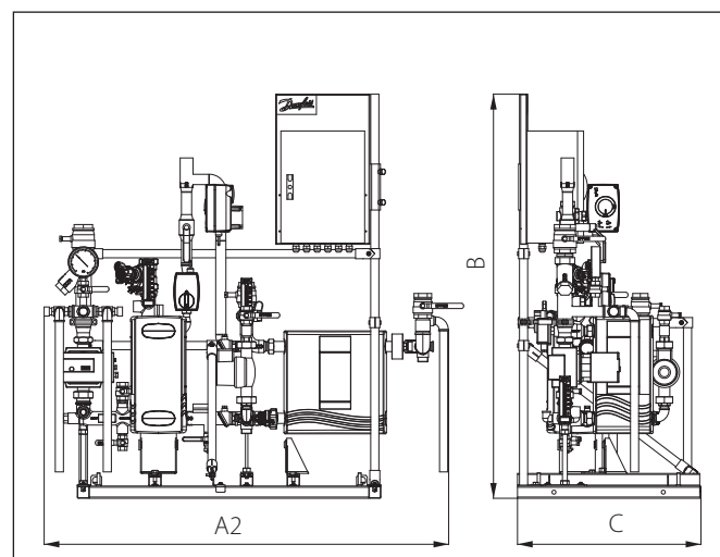
Rys. 1: Zewnętrzne wymiary węzła DSE FLEX
